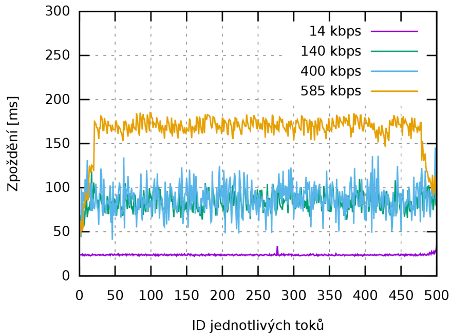
Obr. 3.6: LTE/LTE-A: zpoždění uploadu pro 500 UE a 1 eNodeB [19].
