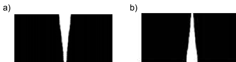
Obr. 3.12 Základní typy tvarů řezných spár: a) V-tvar, b) A-tvar
