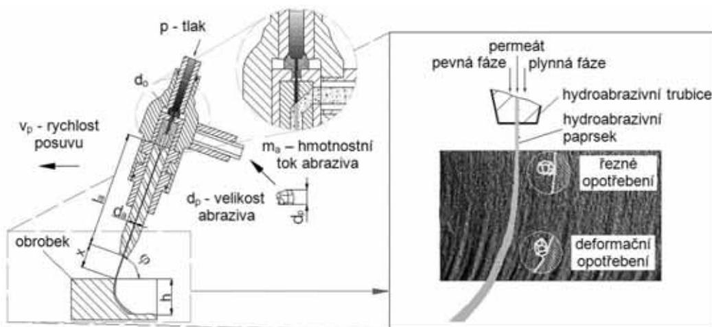
Obr. 3.15 Vliv faktorů AWJ na kvalitu dělicího procesu a jakost topografie povrchu (29)
