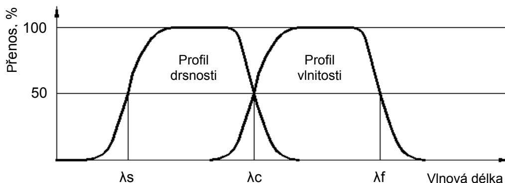
Obr. 4.2 Přenosová charakteristika profilu drsnosti a vlnitosti (34)
