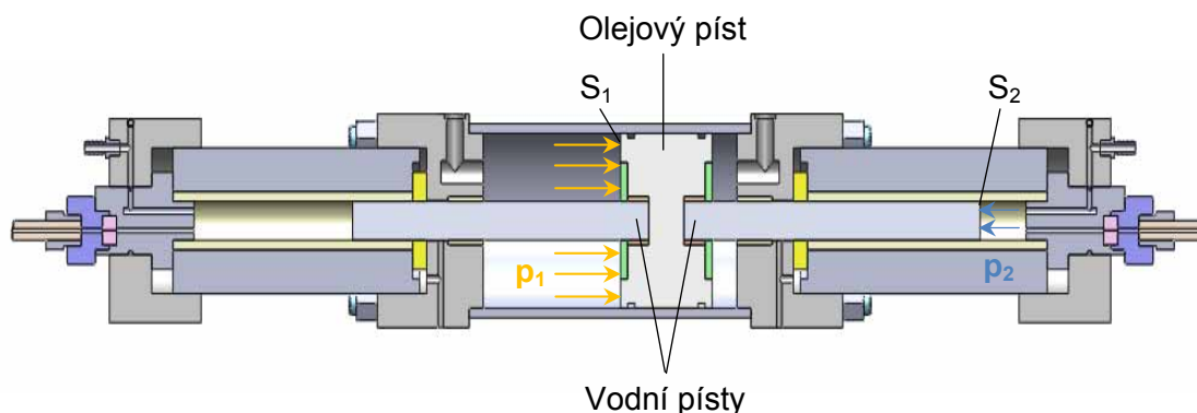
Obr. 3.5 Multiplikátor v řezu (10, 15)
