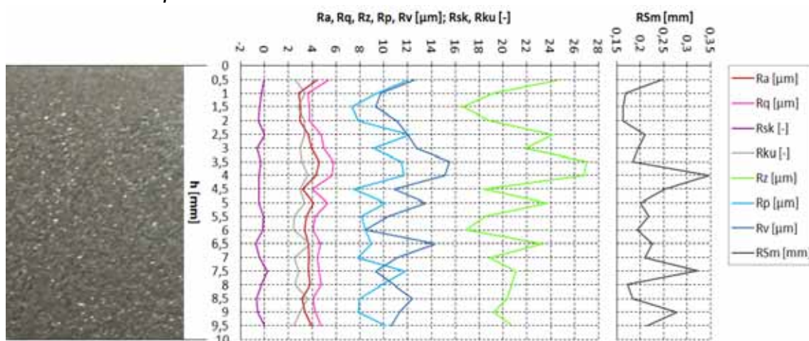
Obr. 5.17 Grafické znázornění závislostí vybraných parametrů profilu drsnosti povrchu na hloubce řezu h při rychlosti posuvu řezné hlavy v_p = 200 \text{ mm/min} (vzorek č. 4)
