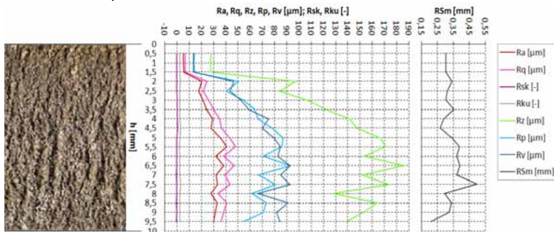
Obr. 5.26 Grafické znázornění závislostí vybraných parametrů profilu drsnosti povrchu na hloubce řezu h při rychlosti posuvu řezné hlavy v_p = 550 mm/min (vzorek č. 2)
