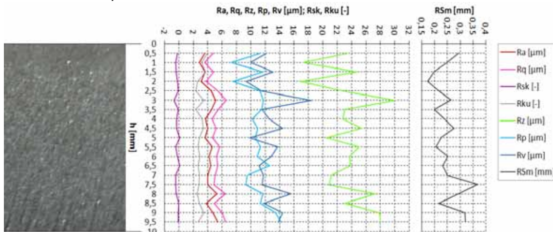
Obr. 5.19 Grafické znázornění závislostí vybraných parametrů profilu drsnosti povrchu na hloubce řezu h při rychlosti posuvu řezné hlavy v_p = 300 mm/min (vzorek č. 6)
