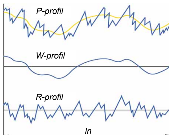
Obr. 4.3 Základní profil a z něho odvozené profily vlnitosti a drsnosti (36)
