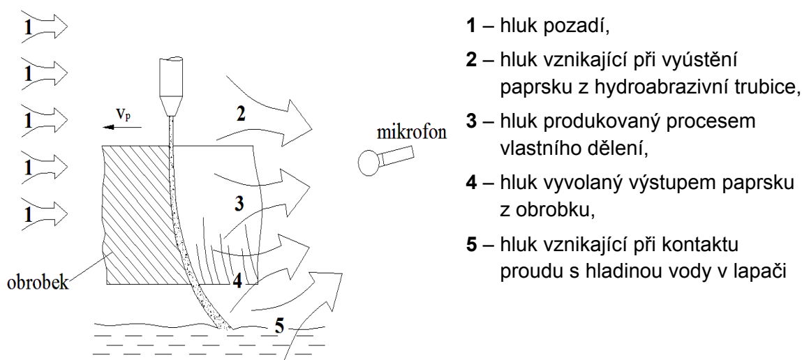
Obr. 3.18 Zdroje emisí akustického tlaku při hydroabrazivním dělení materiálů (2)
