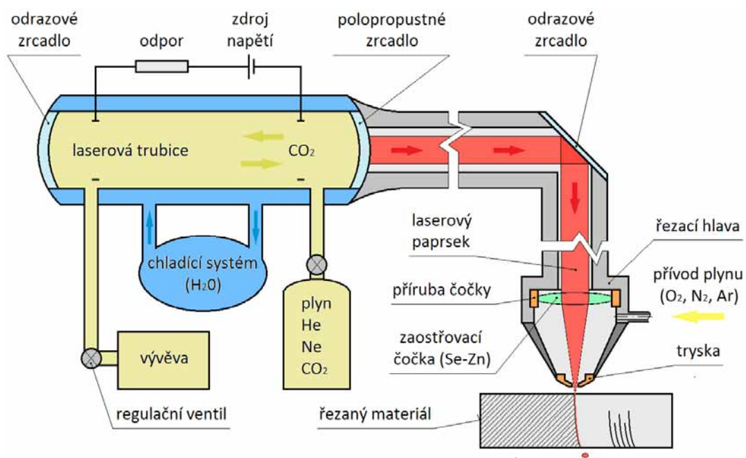
Obr. 5.8 Schematické znázornění principu plynového CO 2 laseru
