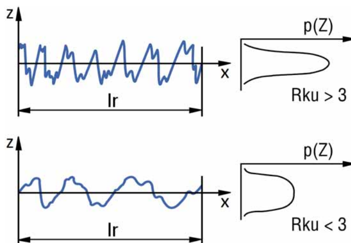
Obr. 4.10 Špičatost posuzovaného profilu Rku
