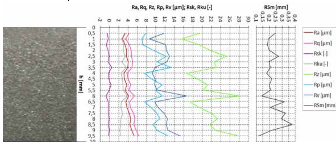
Obr. 5.18 Grafické znázornění závislosti vybraných parametrů profilu drsnosti povrchu na hloubce řezu h při rychlosti posuvu řezné hlavy v_p = 250 \text{ mm/min} (vzorek č. 5)
