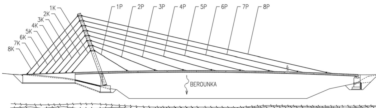
Obr. 5 – značení závěsů
