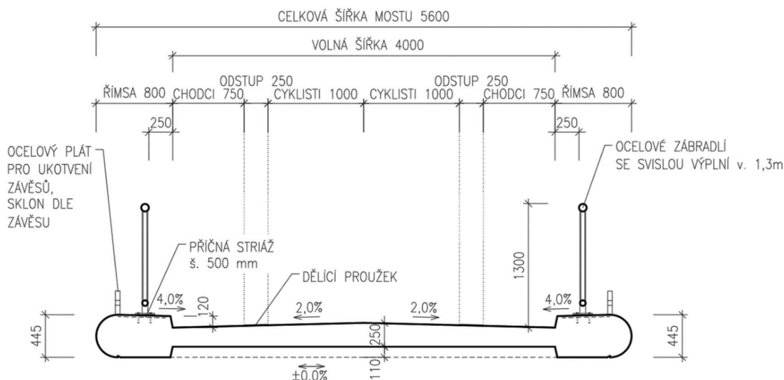
Obr. 3 – příčný řez
