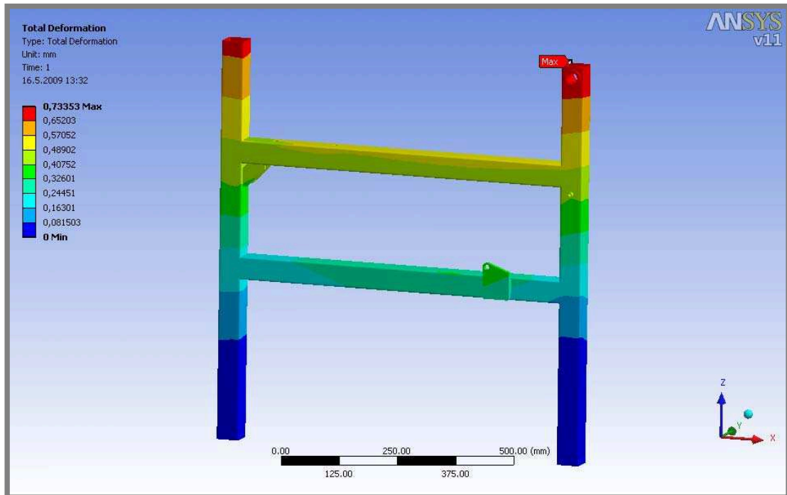
Obr. 6-30 Rám – deformace
