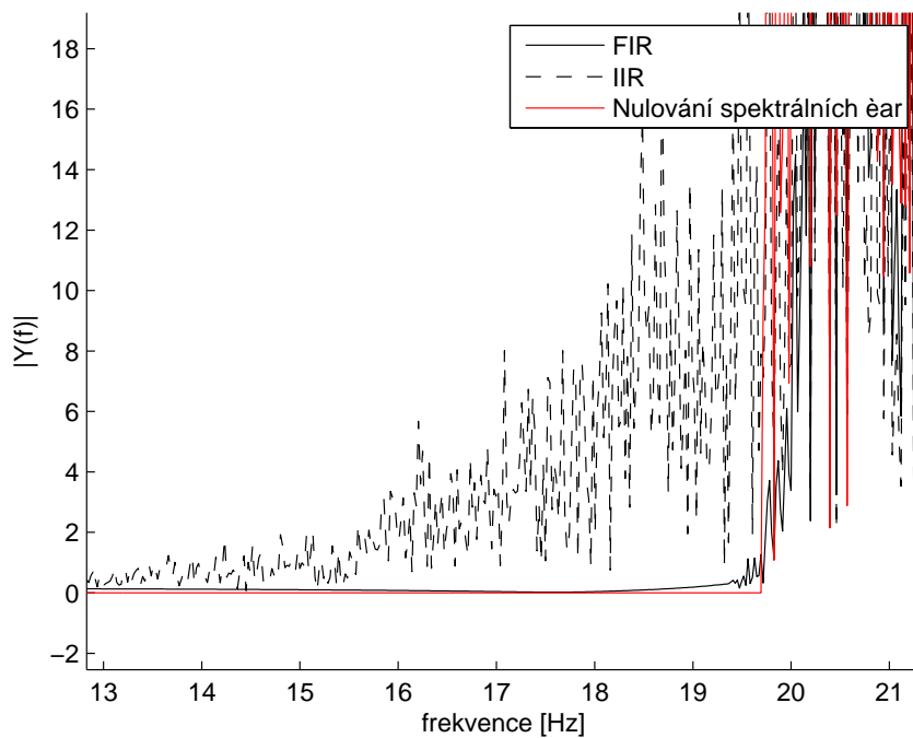
Obrázek 4.2: Srovnání filtrace IIR filtrem, FIR filtrem a nulováním spektrálních čar v frekvenční oblasti kolem mezní frekvence 20 Hz. Nástup IIR filtru je poněkud pomalejší, nepochybně z důvodu nízkého řádu.
