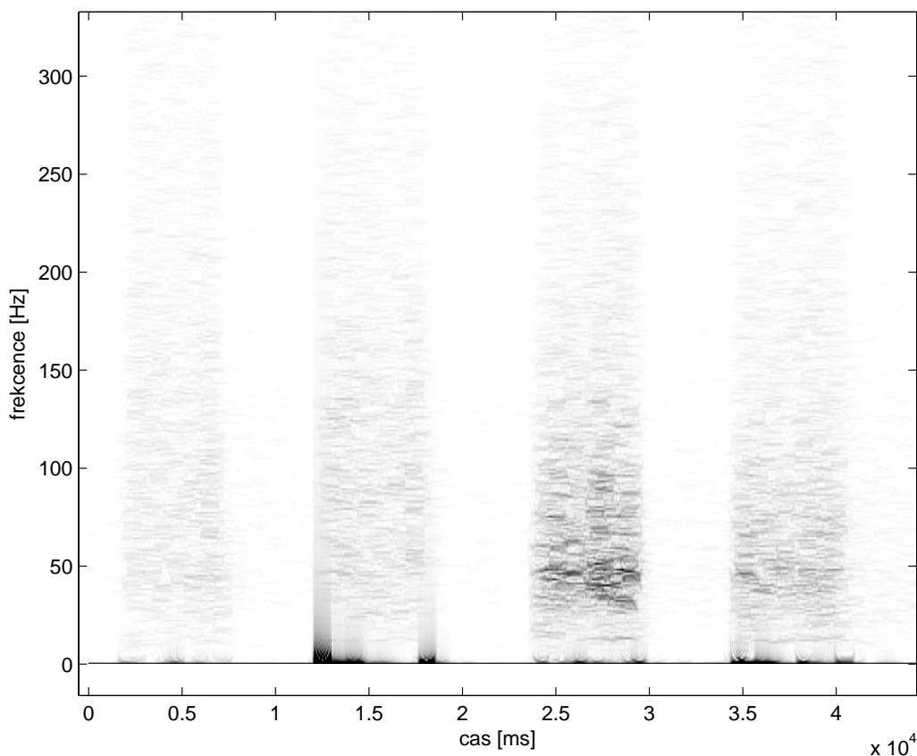
Obrázek 3.3: Normalizovaný spektrogram signálu 1-1-3.mat pomocí STFT. Vzorkovací frekvence 500 Hz. Kolem nulové izolinie si lze povšimnout silného zastoupení driftu a pohybových artefaktů.
