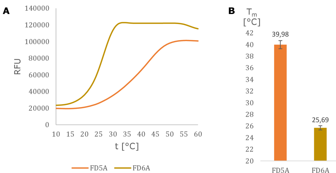
Obr. 31: Výsledky analýzy pomocí DSF (teplotní inkrement 1 ^{\circ}\text{C} za 60 s). A: Průměrné křivky tání FD5A a FD6A (20 \mu\text{g}/\text{ml} ) v PB pufru. B: Porovnání teplot tání FD5A a FD6A s chybovými úsečkami.
