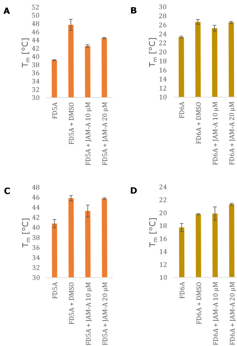
Obr. 33: Průměrné teploty tání FD5A a FD6A (20 \mu g/ml) v PB pufru, s 1 % DMSO, s 10 \mu M JAM-A a 1 % DMSO a s 20 \mu M JAM-A a 1 % DMSO s chybovými úsečkami. A: FD5A, teplotní inkrement 1 °C za 60 s. B: FD6A, teplotní inkrement 1 °C za 60 s. C: FD5A, teplotní inkrement 0,2 °C za 45 s. D: FD6A, teplotní inkrement 0,2 °C za 45 s.
