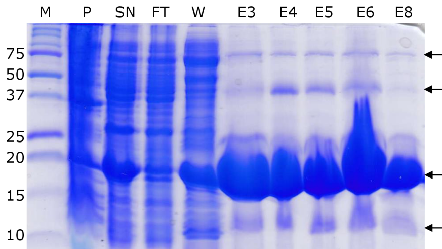
Obr. 12: SDS-PAGE frakcí purifikačního procesu FD5A. Zleva marker molekulových hmotností (M, jednotlivé hmotnosti v kDa jsou přiřazeny vlevo), peleta lyzátu buněčné kultury (P), supernatant lyzátu (SN), frakce na IMAC nezachycených proteinů (FT), proteiny vymyté promývacím pufrém (W), 3. až 6. a 8. eluční frakce (E3-E6, E8).
