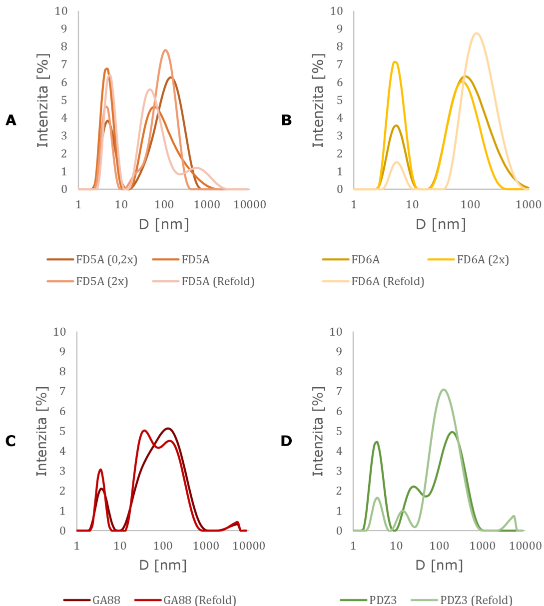
Obr. 26: Intenzitní distribuce (analýza kumulantů autokorelační funkce) jednotlivých proteinů. A: FD5A, koncentrace 0,1 mg/ml (0,2x), 0,5 mg/ml, 1 mg/ml (2x) a refoldovaný 0,5 mg/ml při 20 °C. B: FD6A, koncentrace 0,5 mg/ml a refoldovaný 0,5 mg/ml při 20 °C a 1 mg/ml (2x) při 4 °C. C: GA88, koncentrace 0,5 mg/ml a refoldovaný 0,5 mg/ml při 20 °C. D: PDZ3, koncentrace 0,5 mg/ml a refoldovaný 0,5 mg/ml při 20 °C.
