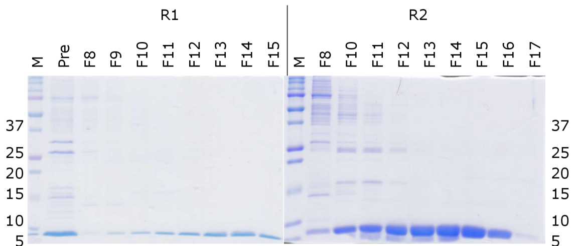
Obr. 23: SDS-PAGE frakcí prvních separací G_A88 pomocí SEC. Zleva marker molekulových hmotností (M, jednotlivé hmotnosti v kDa jsou přiřazeny vlevo), následuje vzorek před SEC o koncentraci 1 mg/ml (Pre) a frakce první (R1) separace: 8. až 15. frakce (F8-R15), marker molekulových hmotností, následují frakce druhé (R2) separace: 8. a 10. až 17. frakce (F8, F10-R17).
