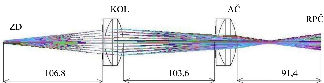
Obrázek 23: Návrh optické soustavy, varianta B. ZD - zdroj, KOL - kolektor, AČ - aperturní čočka, RPČ - rovina polní čočky.
