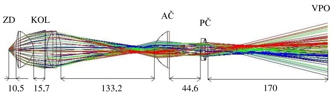
Obrázek 27: Návrh optické soustavy, varianta F. ZD - zdroj, KOL - kolektor, AČ - aperturní čočka, PČ - polní čočka, VPO - vstupní pupila objektivu.
