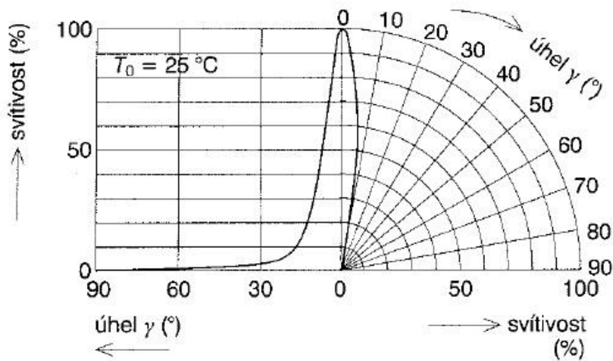
Obrázek 13: Příklad rozložení svítivosti LED v pravouhlých a polárních souřadnicích. Převzato z [20].
