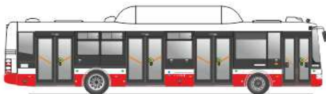
Obrázek 11: Autobus SOR NBG 12 [6]
