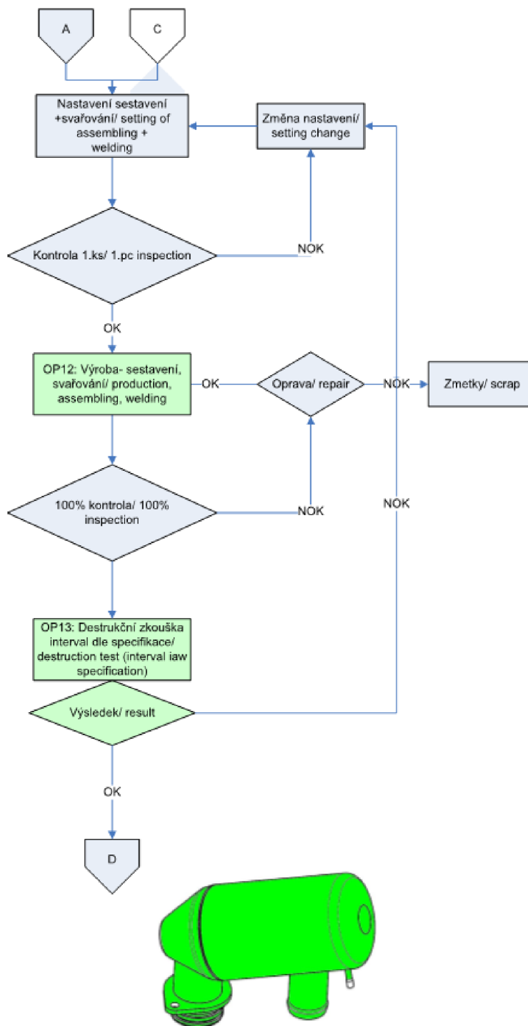
Obrázek 18 Process Flow chart „D“ [2]
