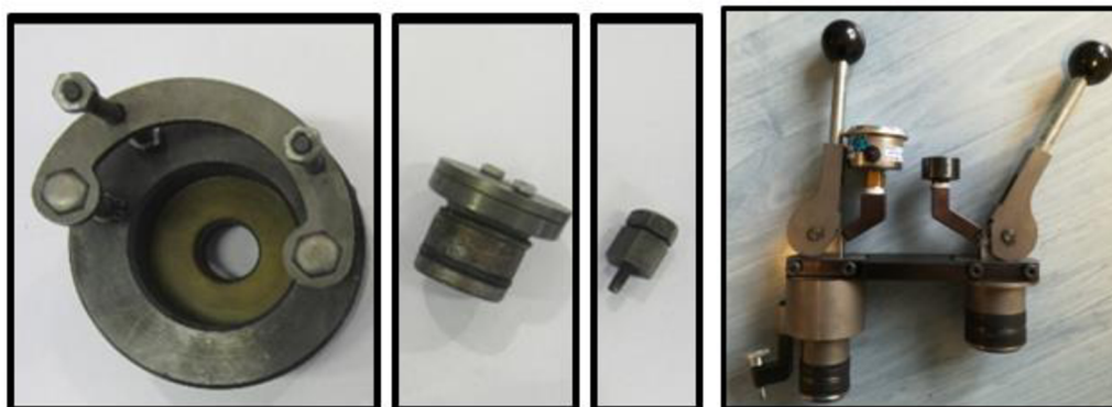
Obrázek 20 Staré přípravky (vlevo) a nový design přípravku (vpravo) [2]
