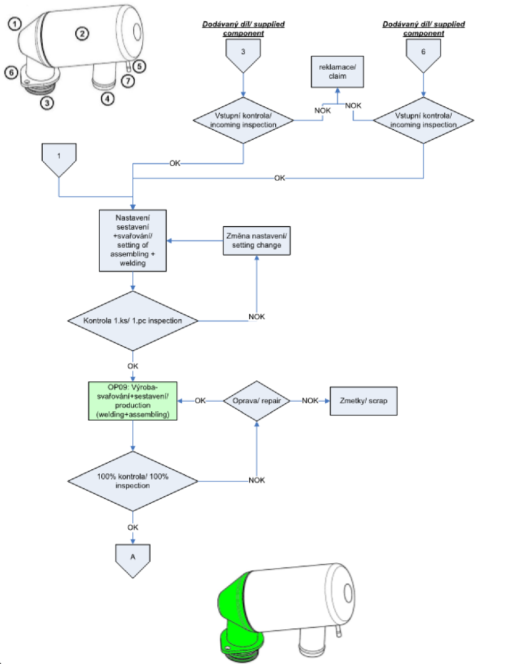
Obrázek 17 Process Flow chart „A“ [2]
