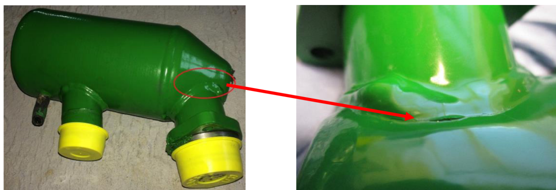
Obrázek 16 Trhlina u svaru na kuželovém dně [2]
