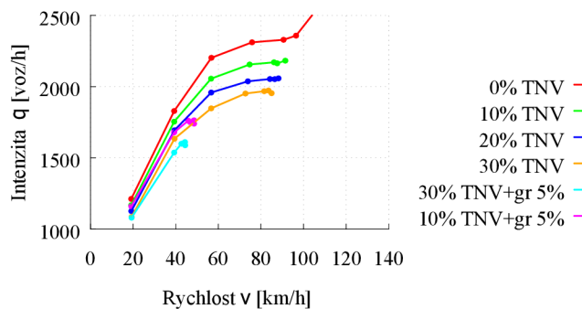
Obř. 7.2: Výředky prvního testu s proměnnou rychlostí a nastavením různého podílu TNV a některé s podélným sklonem komunikace. Jen v programu PTV.
