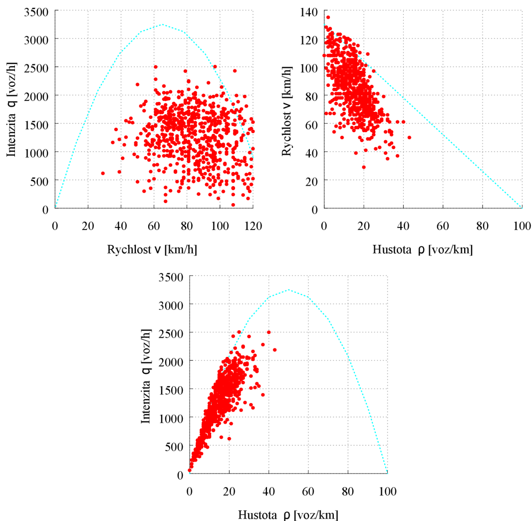
Obr. 7.13: Fundamentální diagramy vzešlé z CA.
