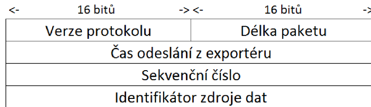
Obrázek 2.5: Hlavička IPFIX paketu
