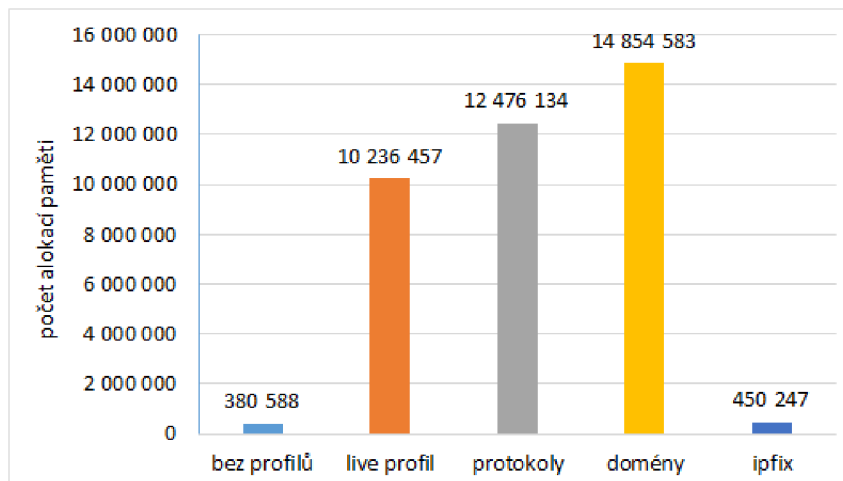
Obrázek 4.6: Počet alokací
