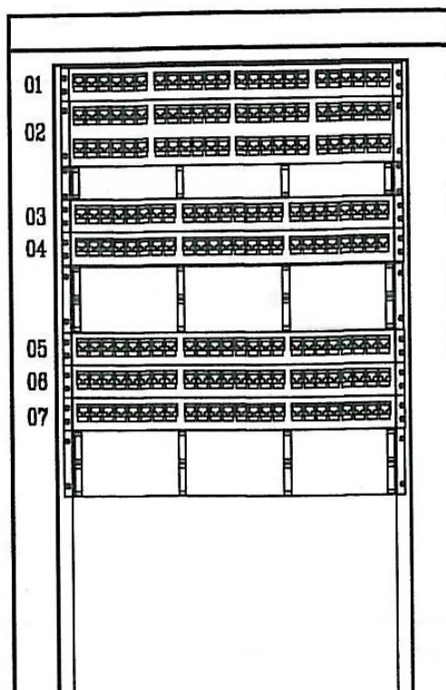
Datový rozvaděč DR1, 42U
