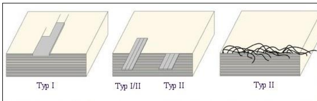
Obr. 10 – Typy delaminací [26]
