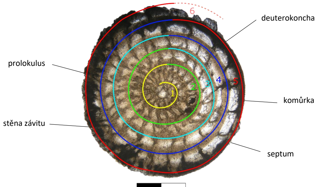
Obr. 24: Popis ekvatoriálního řezu jedincem rodu Nummulites od Březůvek a barevné znázornění závitů. Délka měřítka 1 mm.
