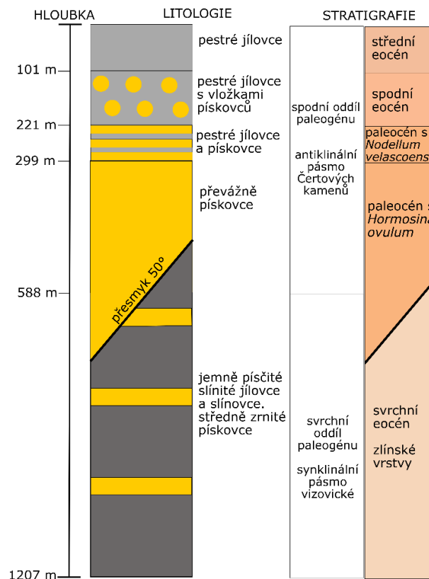
Obr. 7: Stratigraficko-litologický profil vrtu Březůvky-1 (Menčík, Pesl 1964 - upraveno).
