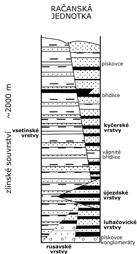
Obr. 4: Litologické schéma zlínského souvrství (Picha a kol. 2006 - upraveno).
