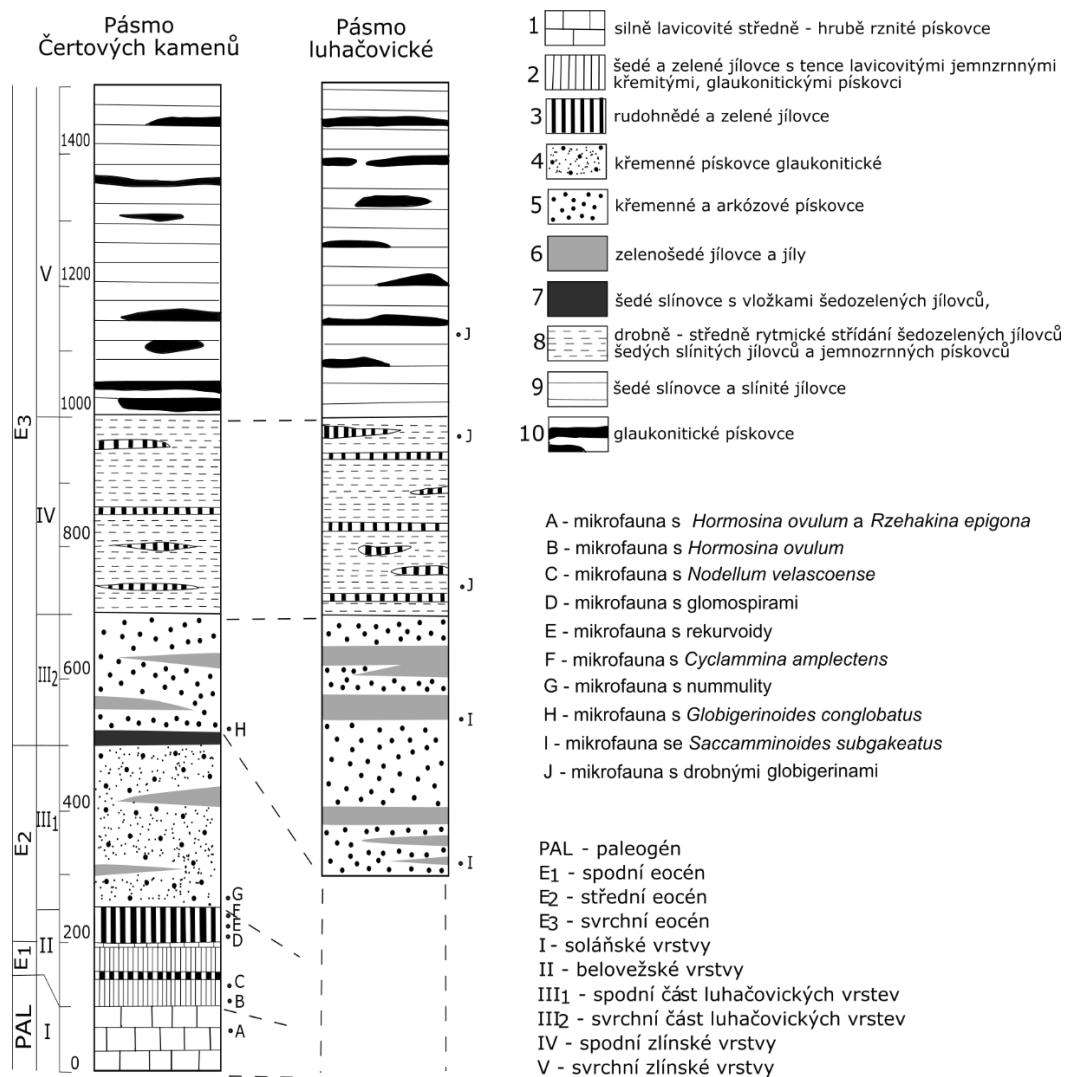
Obr. 9: Litologicko-stratigrafický profil pásma Čertových kamenů a luhačovickým (Menčík, Pešl 1964 - upraveno).
