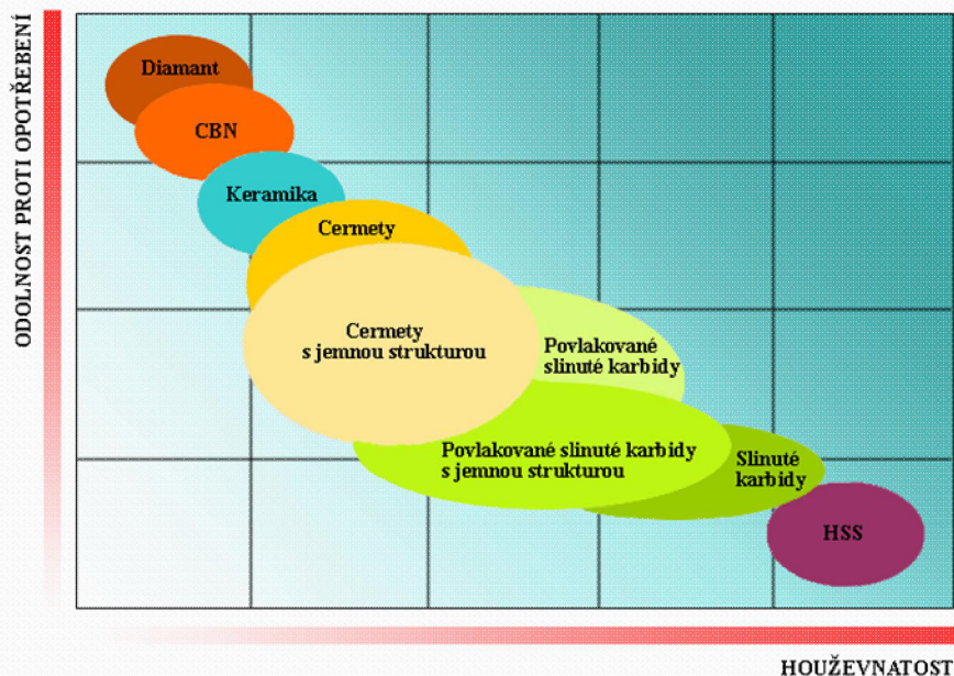
Obrázek 3-10 Řezné materiály a jejich houževnatost s odolností opotřebení 6
