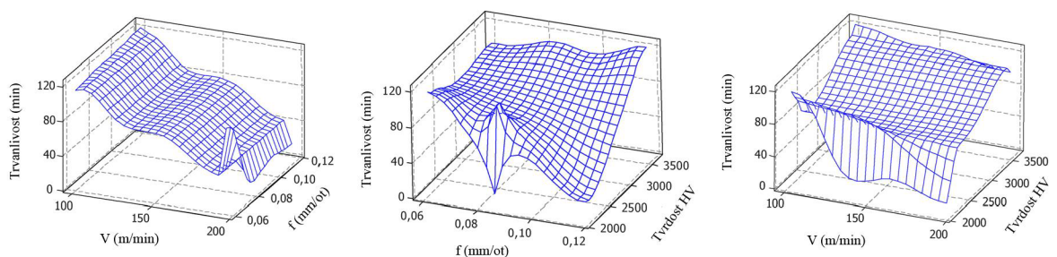
Obrázek 3-2 Trvanlivosti řezné keramiky v různých závislostech 19
