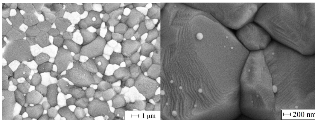
Obrázek 1-9 Mikrostruktura \text{Al}_2\text{O}_3\text{-MgO} vzorků; (vlevo) 80 nm MgO, (vpravo) 80 nm MgO s 30.000 zvětšení 7
