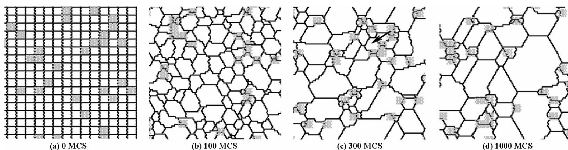
Obrázek 1-5 Simulovaný vývoj struktury materiálu \text{Al}_2\text{O}_3/10\%\text{SiC} metodou Monte Carlo ( 1MCS = 250 000 pc výpočtů ) 18
