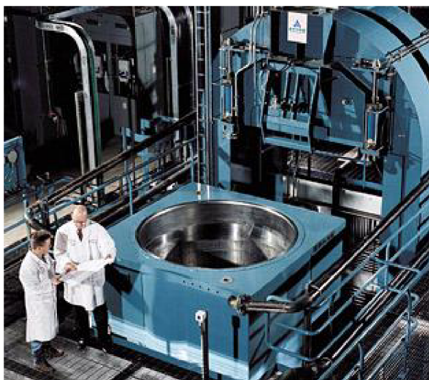
Obrázek 1-3 HIP (Hot Isostatic Press) zařízení od firmy Avure 31
