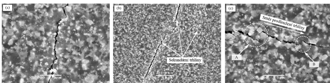
Obrázek 1-4 zamezení trhlin whiskery a) trhlina b) větvení trhliny c) přemostění trhliny 24
