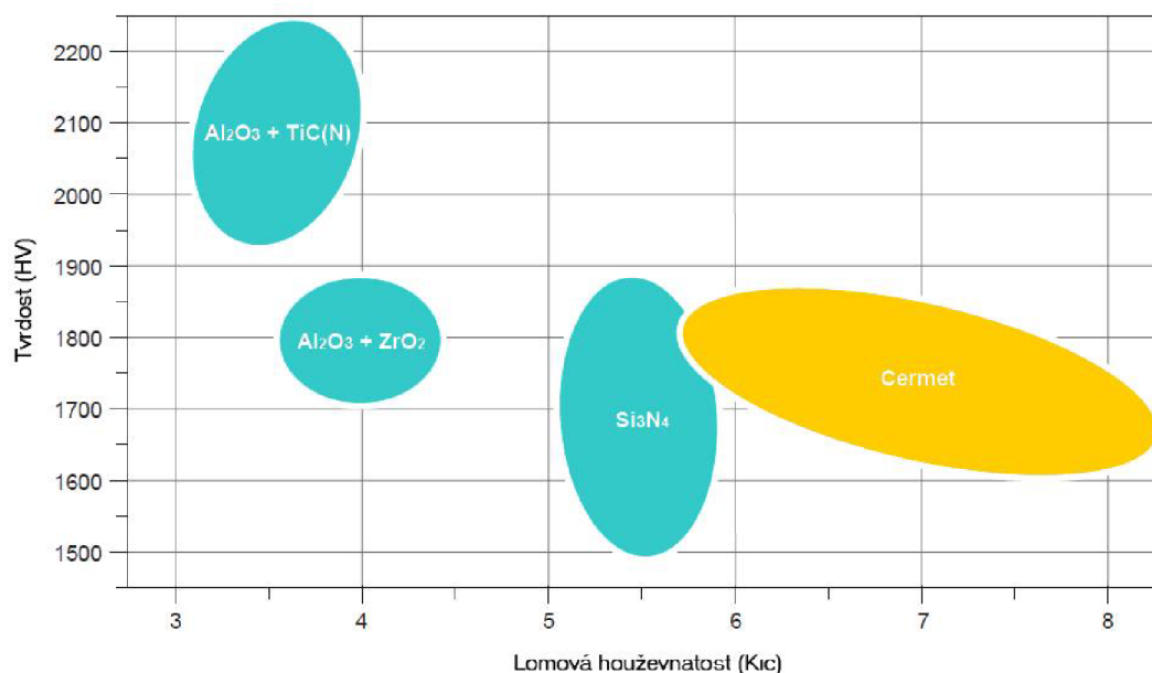
Obrázek 1-10 Srovnání mechanických vlastností jednotlivých keramických materiálů 35
