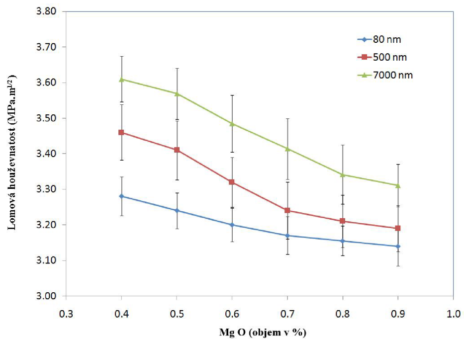
Obrázek 1-11 Ukázka závislosti objemu částic MgO v \text{Al}_2\text{O}_3 a lomové houževnatosti pro velikosti zrn 80,500,7000nm 7
