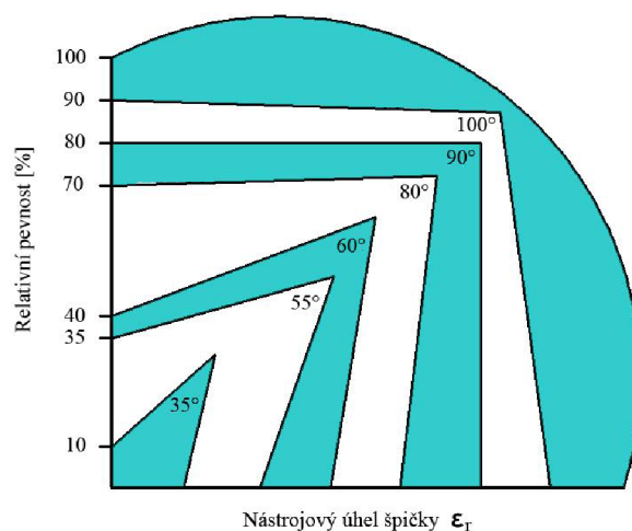
Obrázek 3-6 Relativní pevnost keramické VBD v závislosti na nástrojovém úhlu špičky 30
