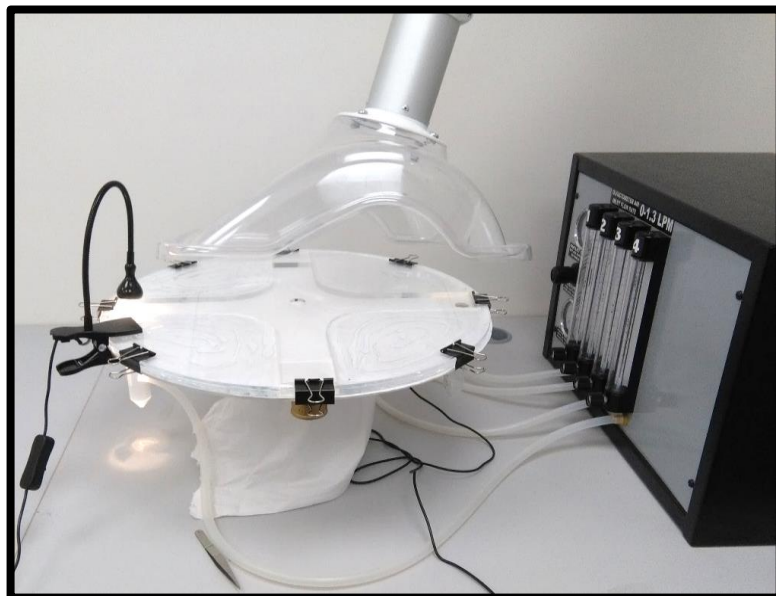
Obr. č. 1: Olfaktometr s uzavřenou kruhovou arénkou, před provedením experimentu 1A. (Majerová ©2019).
