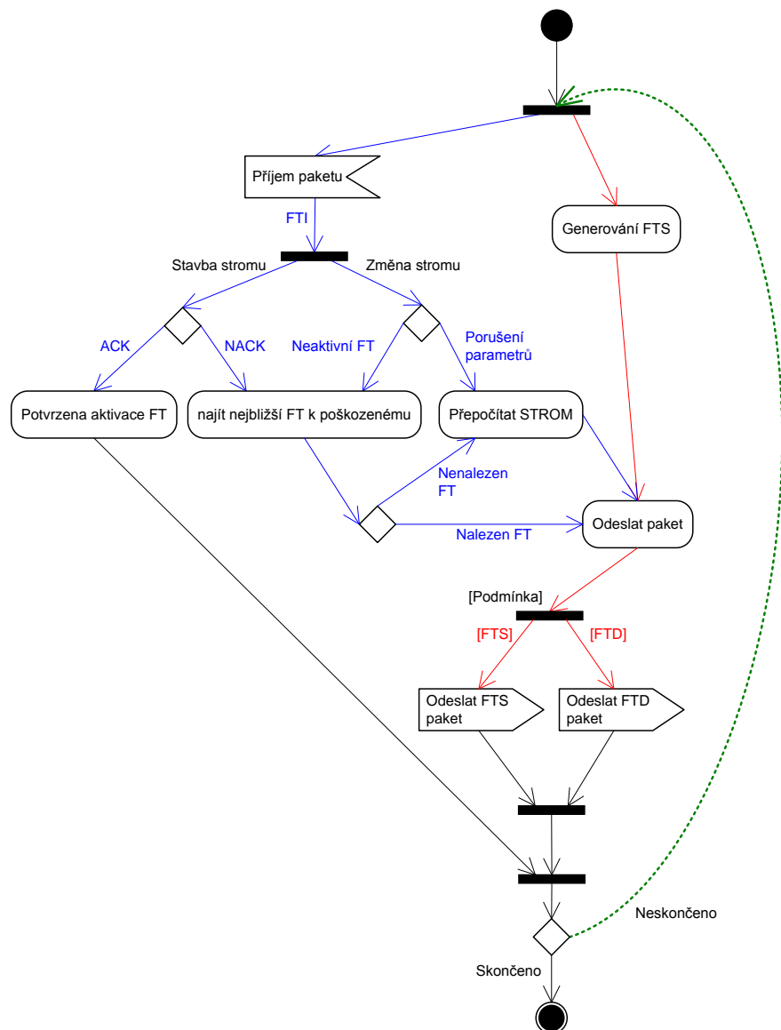
Obr. 4.9 - Stavový diagram FTM
