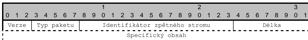
Obr. 2.11 - Hlavička všech paketů TTP
