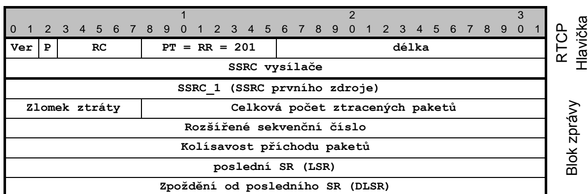
Obr. 2.2 - Struktura informačního paketu RTCP posílaného k vysílači
