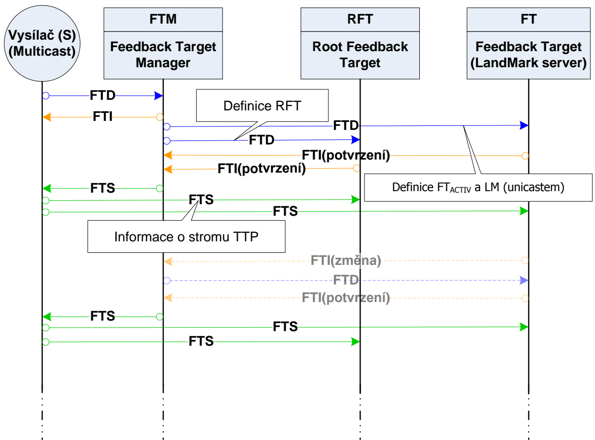
Obr. 4.3 - Sestavení hierarchického stromu zpětného kanálu
