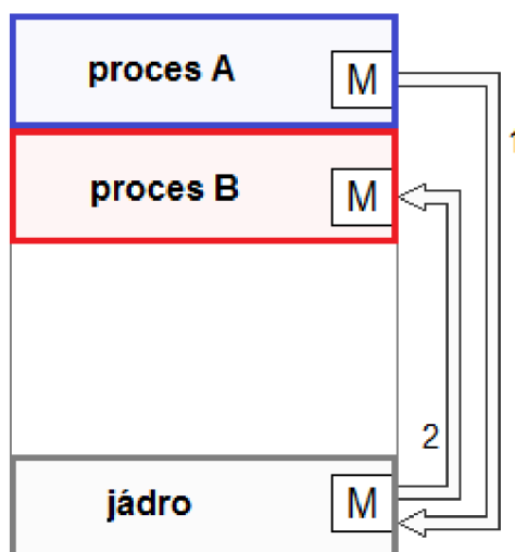
Obrázek 3.1: Ukázka posílání zprávy z procesu A přes jádro procesu B.
