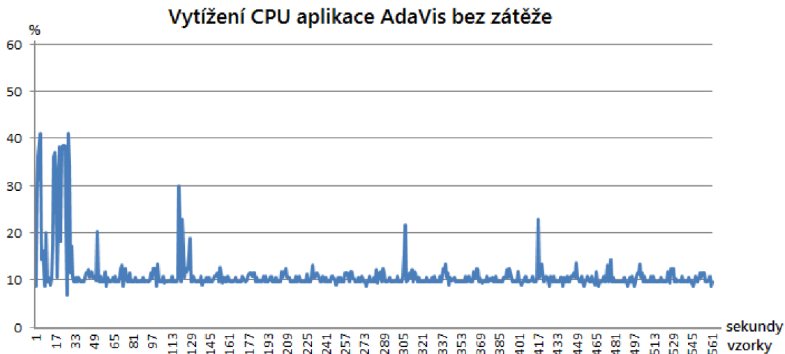
Obrázek 5.4: Vytížení CPU aplikací AdaVis bez zpracovávání vstupních dat.
