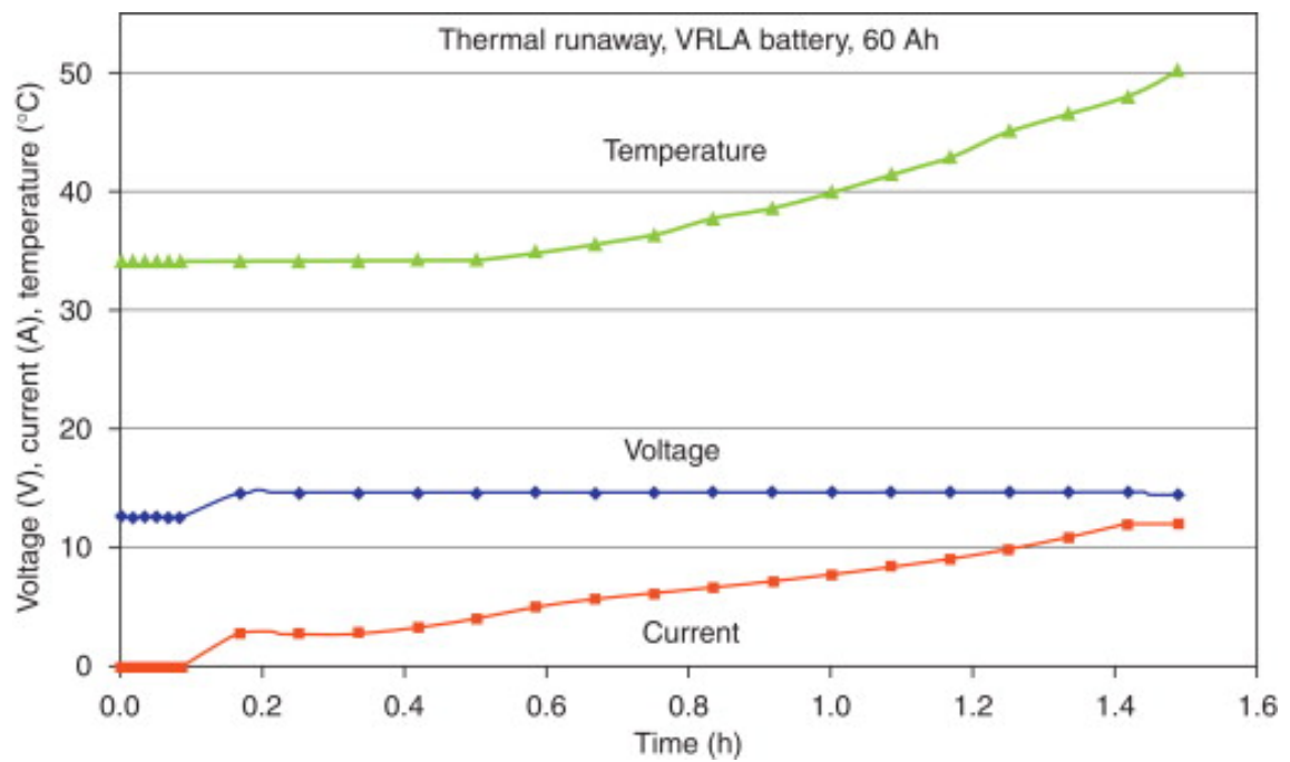
Obr. 2.2: Charakteristiky teploty, proudu a napětí při nabíjení CV [22]
