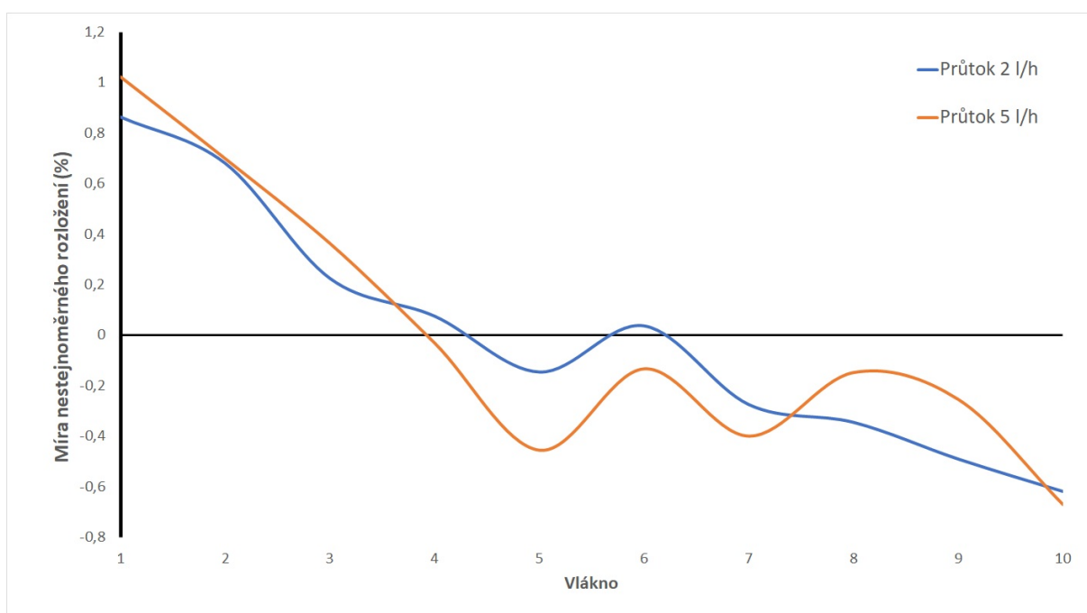
Obr. 5.12: Míra nesterjnoměrného rozložení průtoku ve vláknech pro variantu (a)
