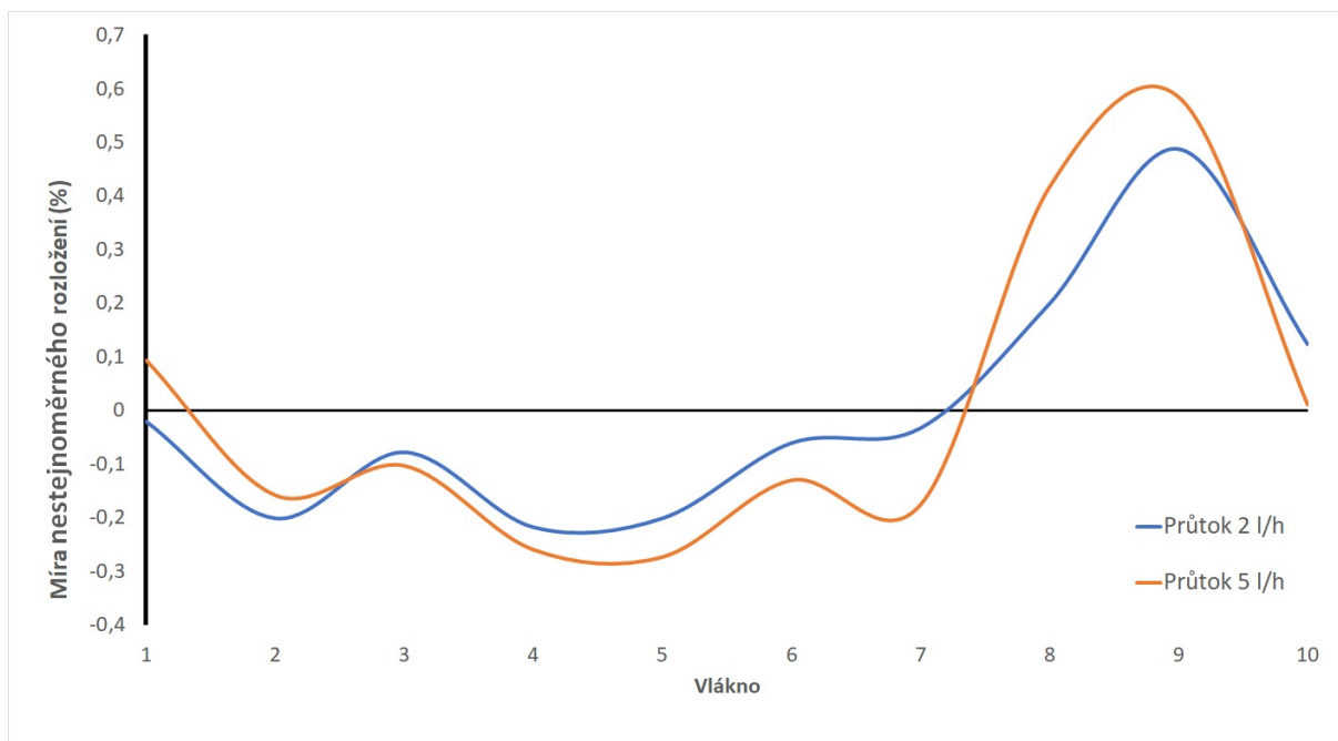
Obr. 5.12: Míra nesterjnoměrného rozložení průtoku ve vláknech pro variantu (a)
