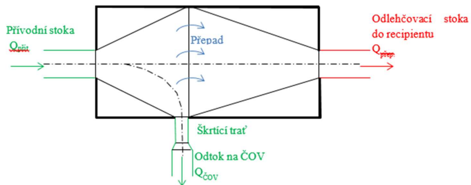
Obrázek 10: Odlehčovací komora s přepadem přímým s kolmou hranou a se škrticí trati
