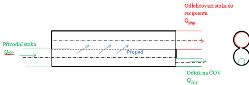
Obrázek 16: Odlehčovací komora s horizontální dělicí stěnou s odtokem do recipientu
