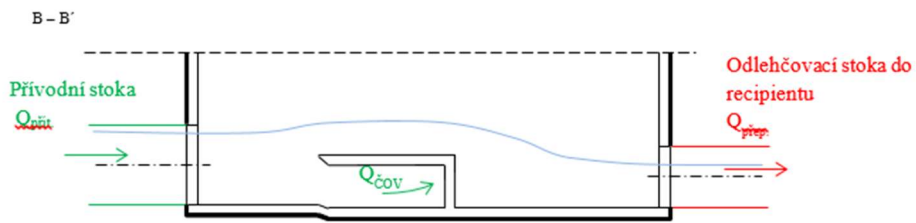
Obrázek 15: Odlehčovací komora s horizontální dělicí stěnou s odtokem na ČOV
