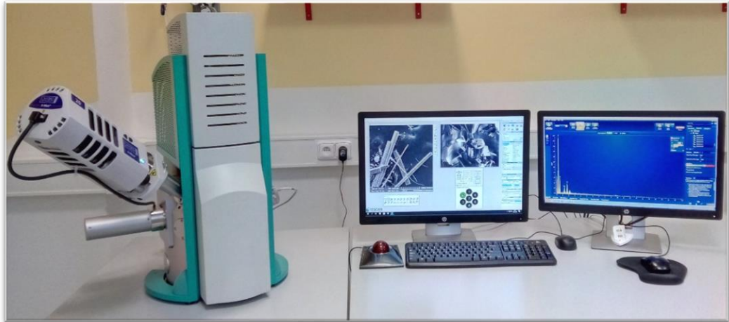
Obrázek 46: Elektronový mikroskop TESCAN VEGA 3 s EDX detektorem (autor)
