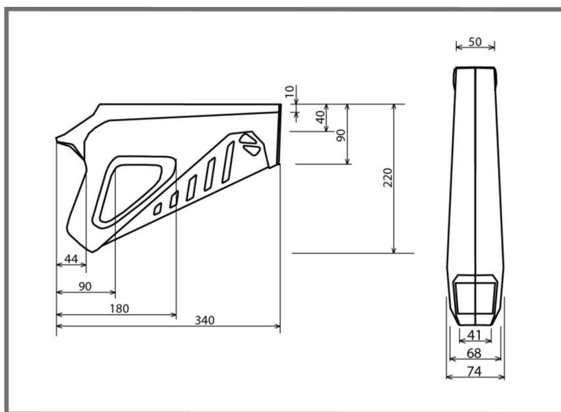
Obr. 5-8 Rozměry zbraně
