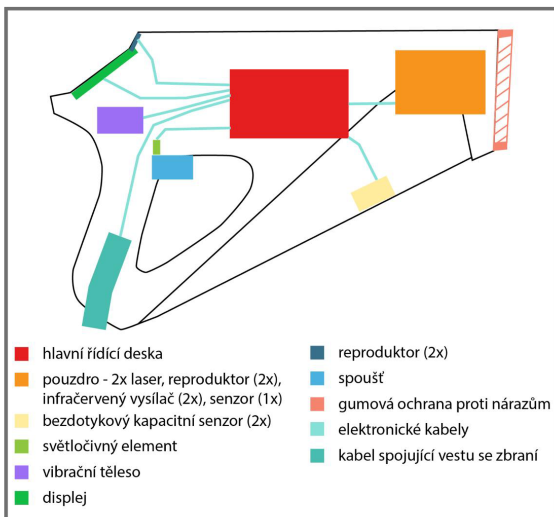
Obr. 5-6 Vnitřní komponenty
