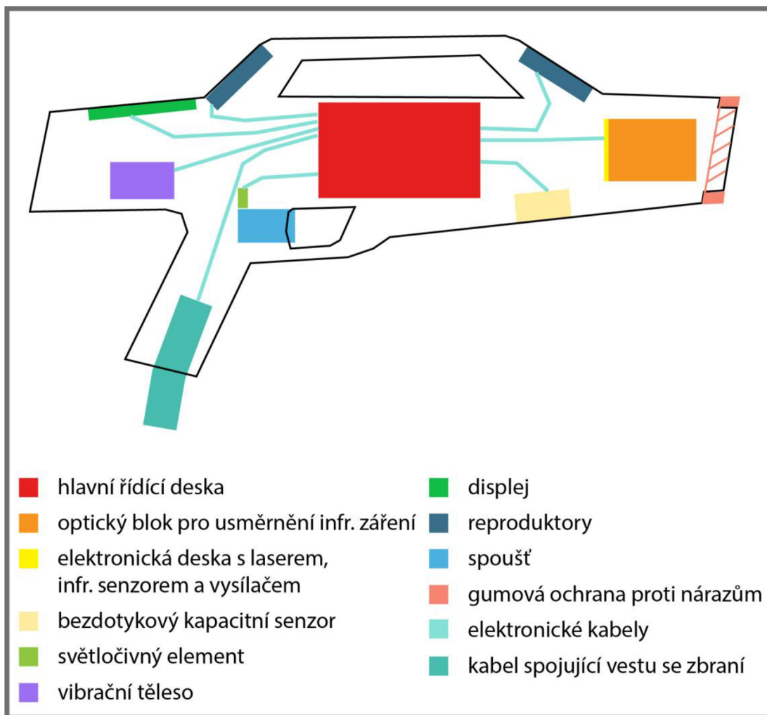
Obr. 1-5 Vnitřní komponenty
