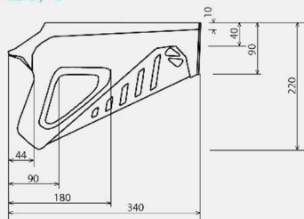
Rozměry 1:2
