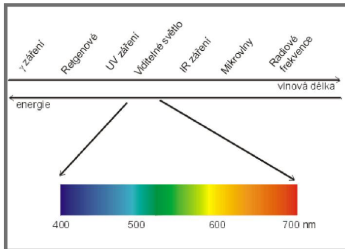
Obr. 1-6 Elektromagnetické spektrum [15]
