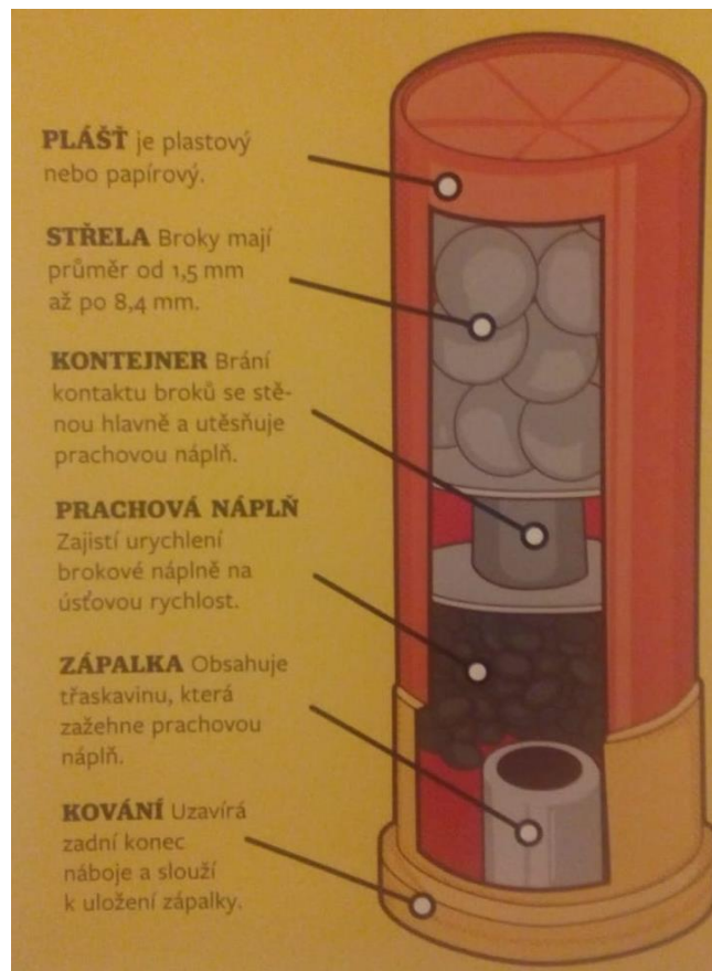
Obr. č. 3 Průřez brokového náboje (Petzal & Bourjaily, 2013)
