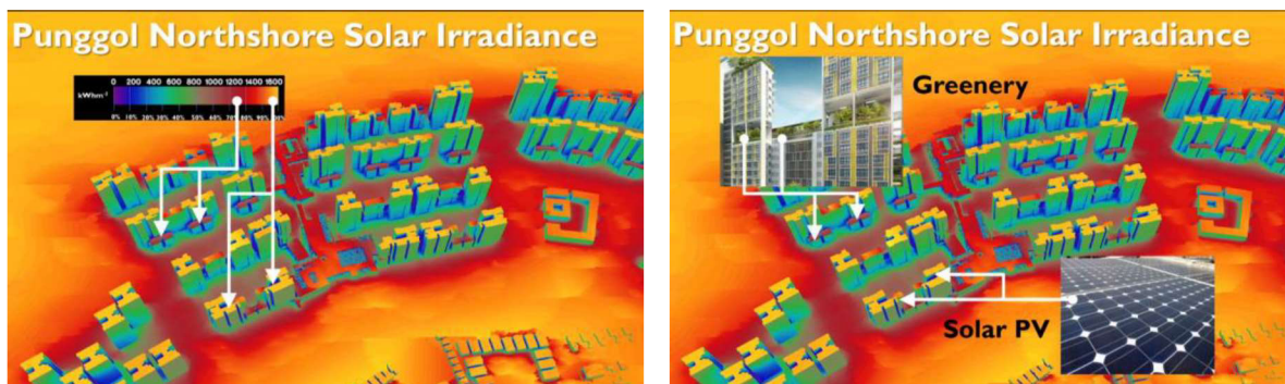
Obr. 4 Simulácia dopadu slnečného žiarenia [6]
