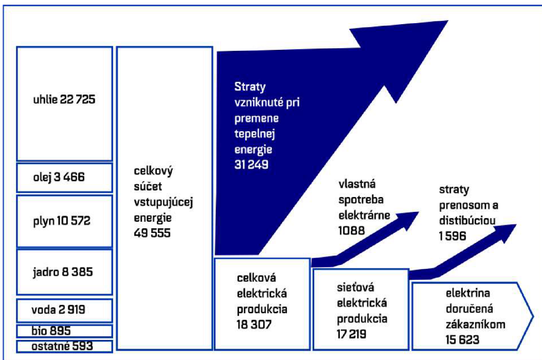
Obr. 6 Znáznornenie celosvetové straty energie na úrovni 68% predtým, ako sa dostane k spotrebiteľovi. [11]
