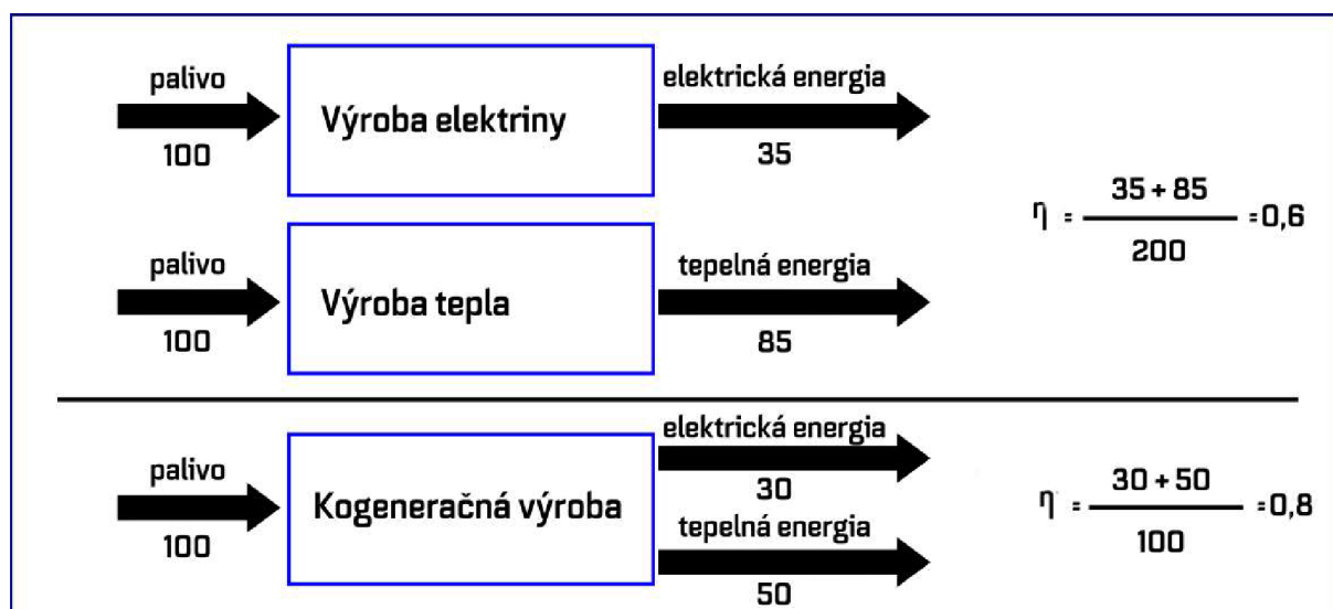
Obr. 8 Porovnanie účinností samostatnej a kombinovanej premeny energie. [10]
