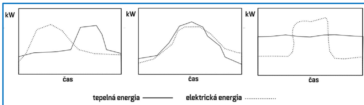
Obr. 12 Závažové krivky [12], [15]
