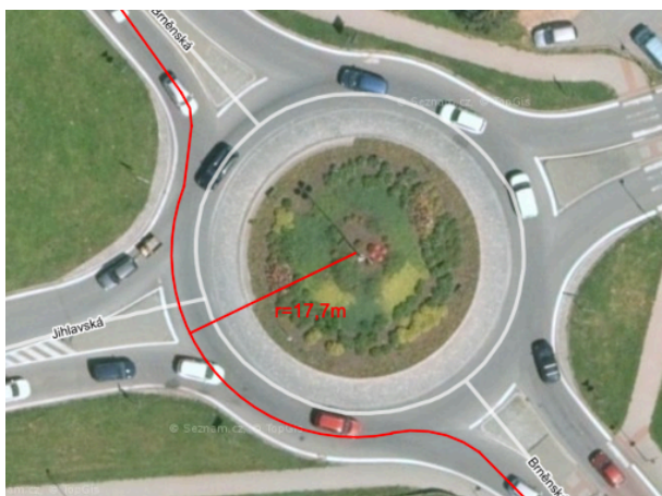
Obrázek 2.4 Kruhový objezd [1]
