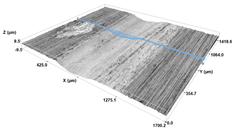
Opotřebení povrchu vzorku H13-N-nav-Rc44 (vlevo – kulička, vpravo – povrch vzorku) při 300 °C
