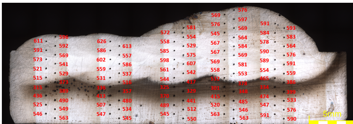
Obr. 3.3 Naměřené tvrdosti v příčném řezu návaru – stav po navaření ( Cronitex Rc 44) Teplota předehřevu při navařování: cca 320 °C
