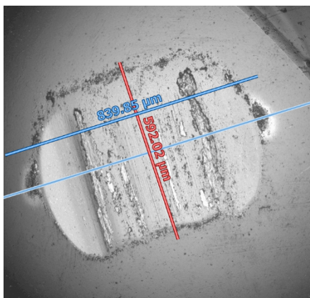
Opotřebení povrchu vzorku H13-N-nav-Rc44 (vlevo – kulička, vpravo – povrch vzorku) při 400 °C
