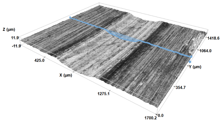
Opotřebení povrchu vzorku H13-N-nav-Rc44 (vlevo – kulička, vpravo – povrch vzorku) při 400 °C
