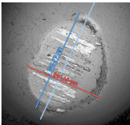
Opotřebenění povrchu vzorku H13-nav-Rc44 (vlevo – kulička, vpravo – povrch vzorku) při 500 °C
