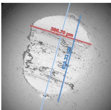
Opotřebení povrchu vzorku H13-N-nav-Rc44 (vlevo – kulička, vpravo – povrch vzorku) při 300 °C
