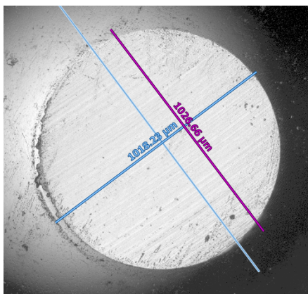
Opotřebení povrchu vzorku H13-N-nav-Rc44 (vlevo – kulička, vpravo – povrch vzorku) při RT
