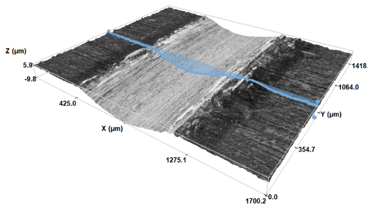
Opotřebenění povrchu vzorku H13-nav-Rc44 (vlevo – kulička, vpravo – povrch vzorku) při 500 °C
