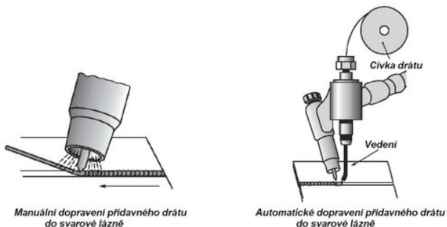
Obr. 2.17a Manuální podávání materiálu [39] Obr. 2.17b Mechanické podávání materiálu [39]
