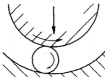
Obr. 2.8a Mechanismus únavového opotřebení(ložisko) [21]
