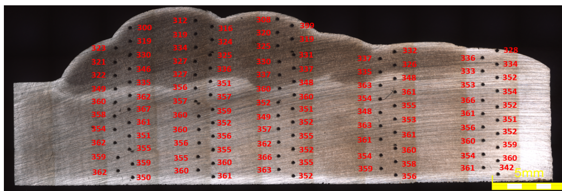
Obr. 3.5 Naměřené tvrdosti v příčném řezu návaru – stav po zakalení a popouštění ( Cronitex Rc 44) Popouštění: při teplotě 570 °C
