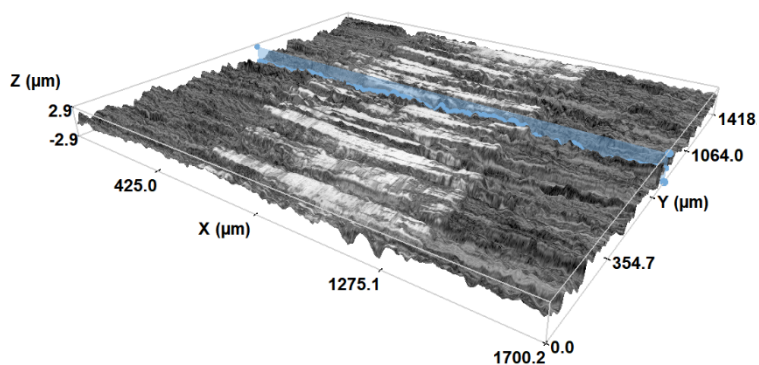
Opotřebení povrchu vzorku H13-N-nav-Rc44 (vlevo – kulička, vpravo – povrch vzorku) při RT
