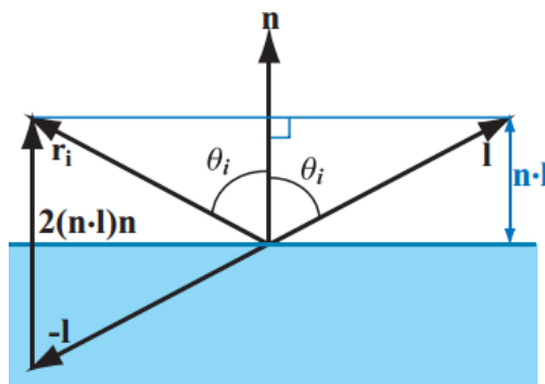
Obrázok 7.8: Nájdenie vektora, ktorý prináša do kamery svetlo odrazené z prostredia. Vektor \mathbf{l} smeruje z miesta dotyku lúča s hladinou do kamery. Vektor \mathbf{n} je normála vodnej hladiny. Vektor \mathbf{r}_i je hľadaný vektor (prevzaté z [6])
