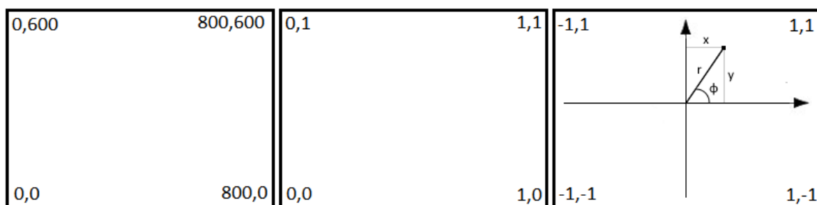
Obrázok 3.4: Príklad prevodu pozície pixelu z window-space (okno má veľkosť 800x600). Pozícia je najprv normalizovaná a následne je transformovaná do klasického kartézského súradnicového systému s počiatkom v strede obrazovky. Z pozície pixelu je možné dopočítať polárne súradnice
