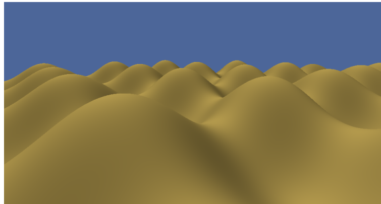
Obrázok 7.1: Vykreslenie výškovej mapy danej funkciou 10\sin(0.1x)\sin(0.1z) . Obrázok je vykreslený naivnou verziou ray marchingu s pevnou dĺžkou kroku. Spôsob výpočtu osvetlenia je vysvetlený v časti 7.2.
