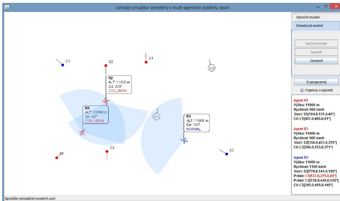
Obrázek 4.8: Okno aplikace při spuštění simulace.
