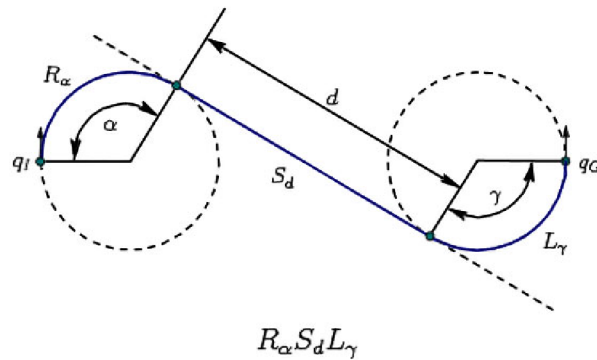
Obrázek 4.7: Příklad sekvence kroků typu RSL [10].
