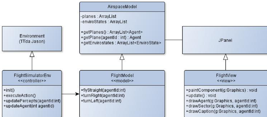
Obrázek 4.3: Diagram tříd simulačního modulu.
