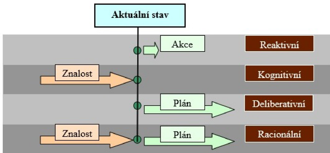
Obrázek 2.3: Dělení agentů [14].
