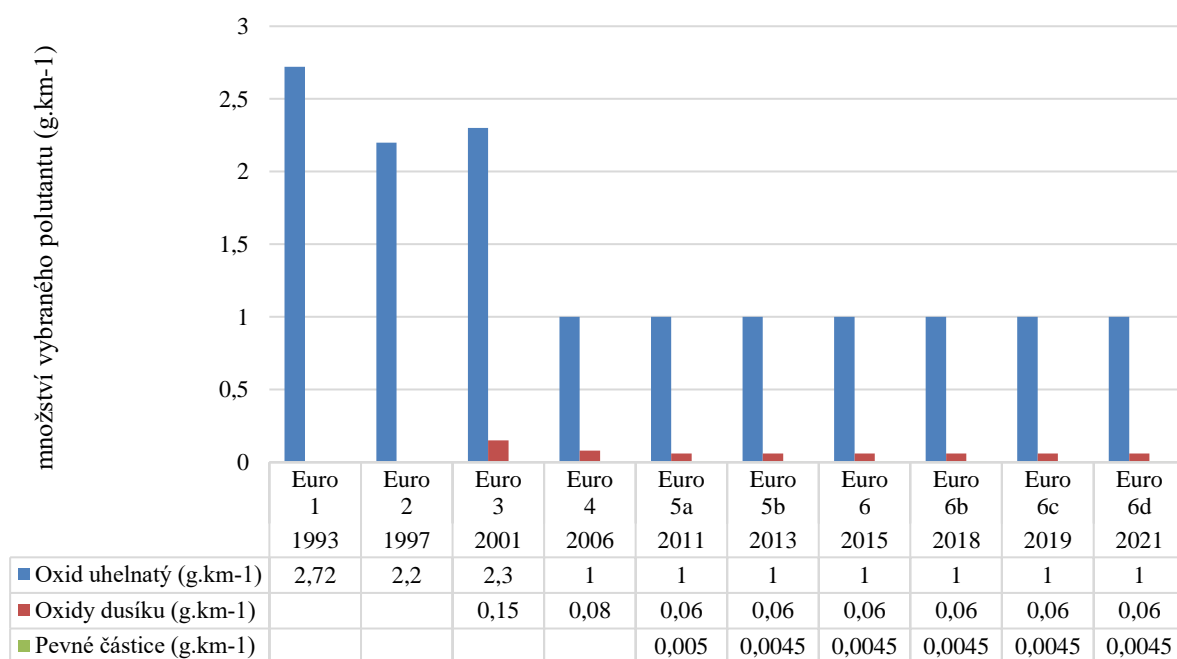
Obr. 11: Zavedené emisní třídy EURO pro benzínové motory [22]
