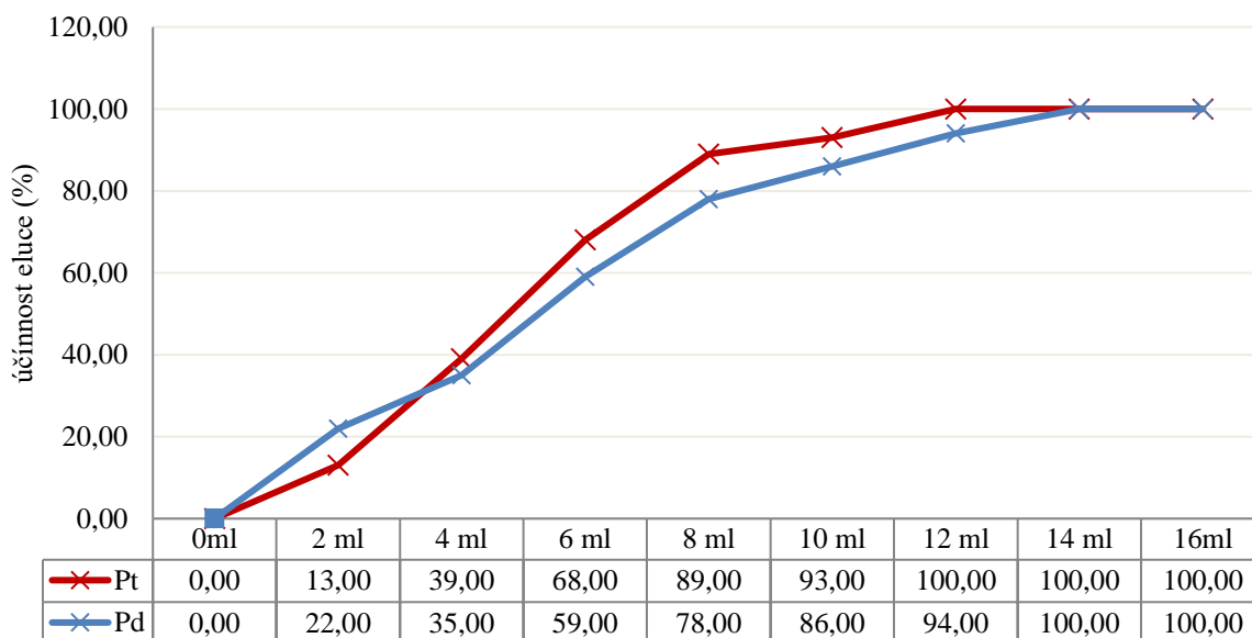
Obr. 58: Účinnost eluce za použití rozpouštědla acetonitrilu na modifikovaný sorbent – SDB
