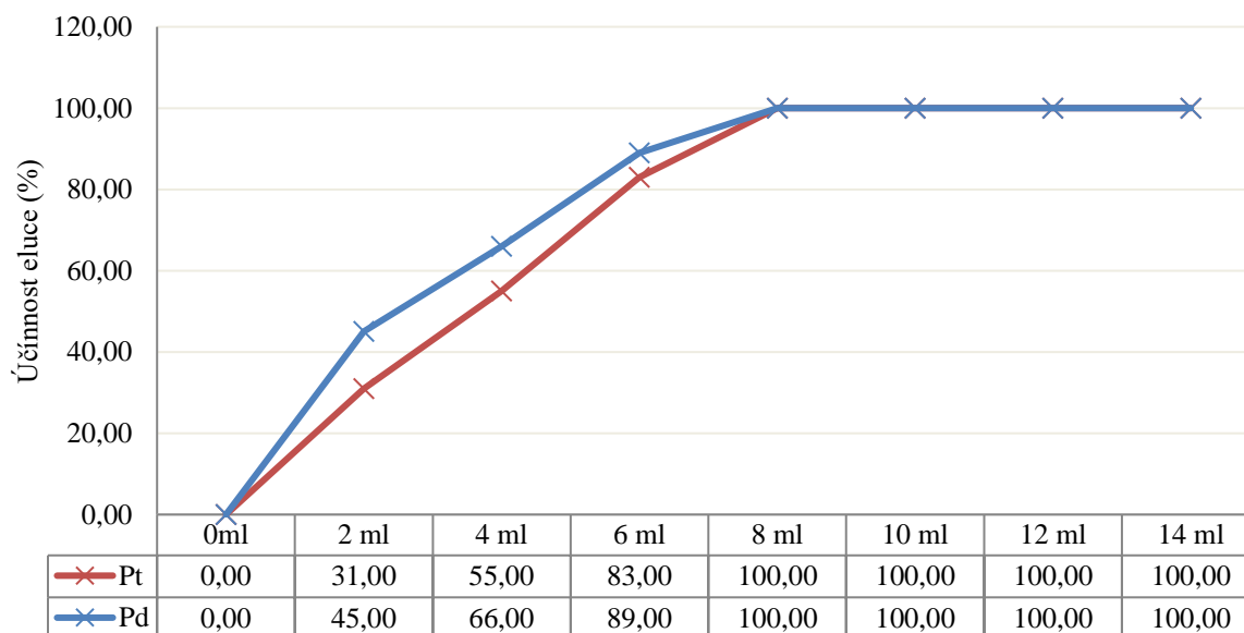
Obr. 50: Účinnost eluce za použití elučního činidla acetonitrilu na modifikovaný sorbent – Silikagel C18
