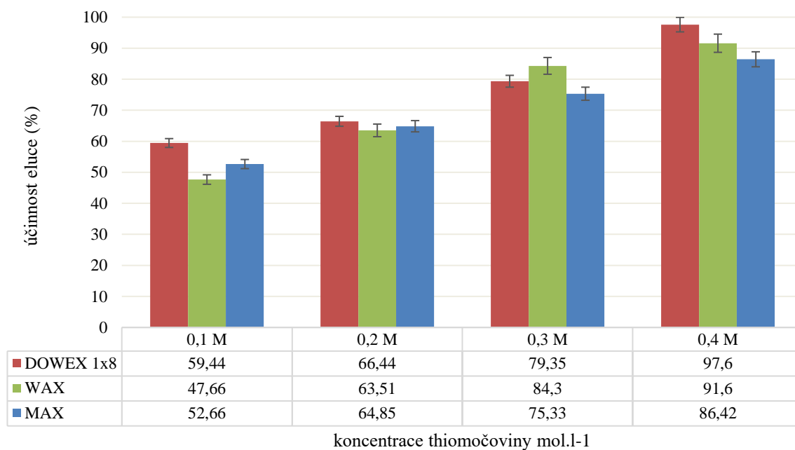
Obr. 63: Vliv koncentrace thiomocoviny na účinnost eluce palladia z aniontoměničových pryskyřic
