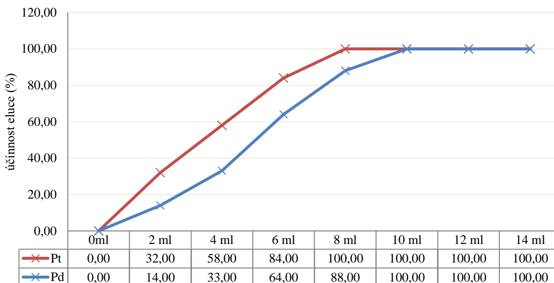
Obr. 56: Účinnost eluce za použití rozpouštědla acetonitrilu na modifikovaný sorbent – Silikagel Si-I
