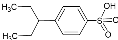
Obr. 38: DOWEX 50W-X8
