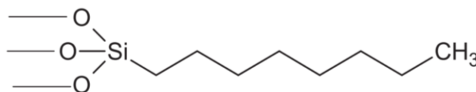
Obr. 33: Silikagel C-8 [122]
