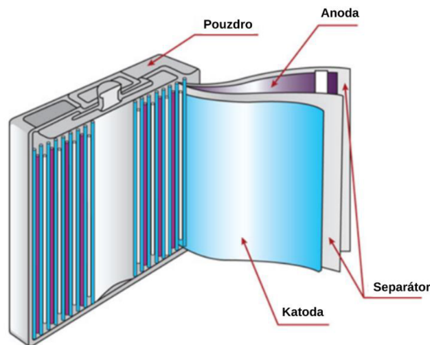
Obr. 11 Složení prizmatického článku, upravené [20]
