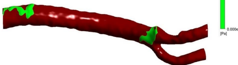
Obrázek 5.19 Kritické oblasti smykového napětí na stěně pro tepnu s 30% stenózou
