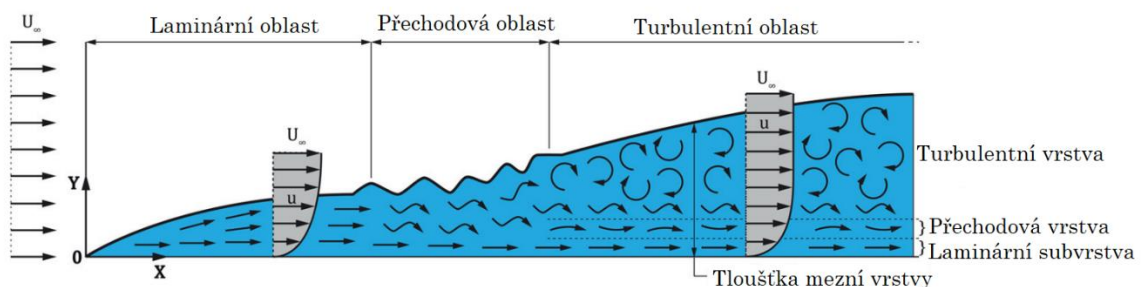
Obrázek 4.1 Typy proudění. Převzato a upraveno z [45]
