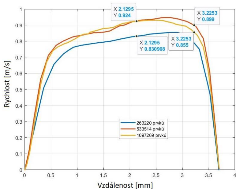
Obrázek 5.7 Porovnání rychlostních profilů na ICA v oblasti za stenózou za použití různých velikostí sítí
