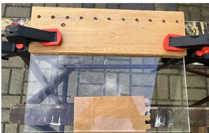
Obrázek 7.1: Vrtání mřížky pomocí šablony (zdroj: autor)
