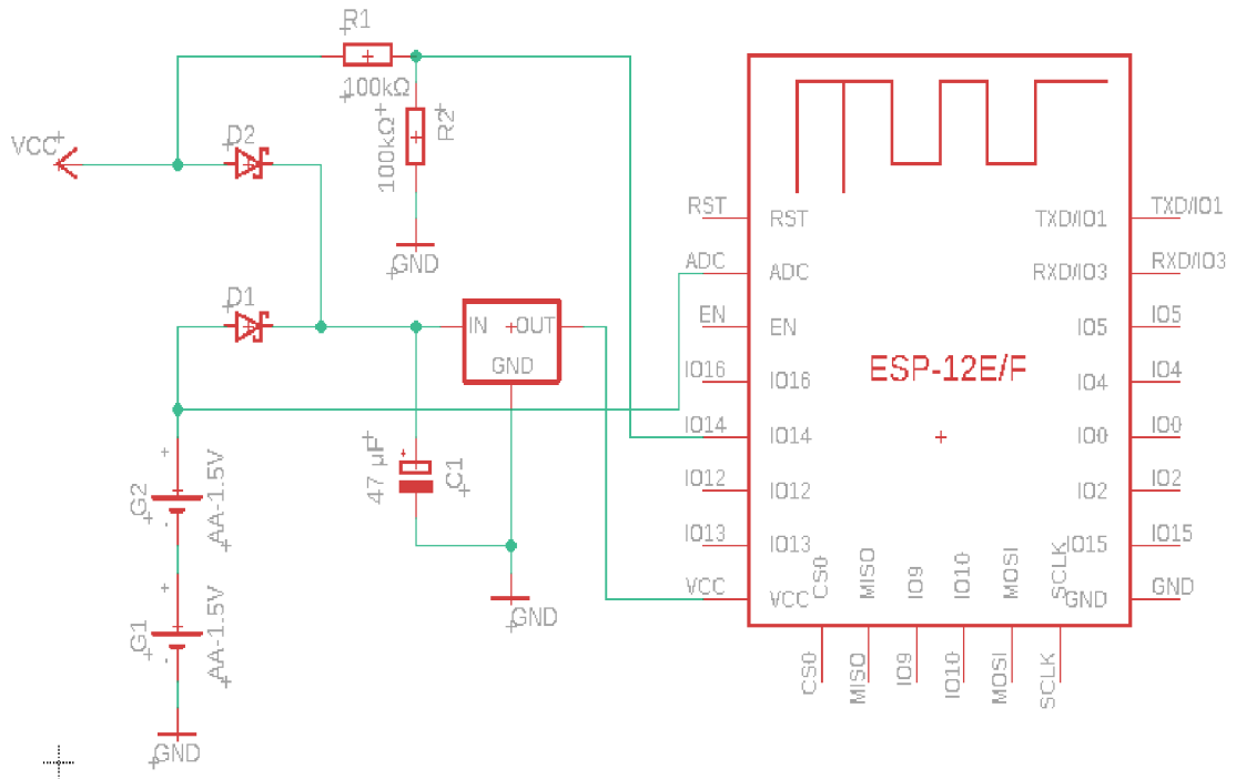
Obr. 5.1: Elektrické schéma zapojení napájení a detekce zdroje
