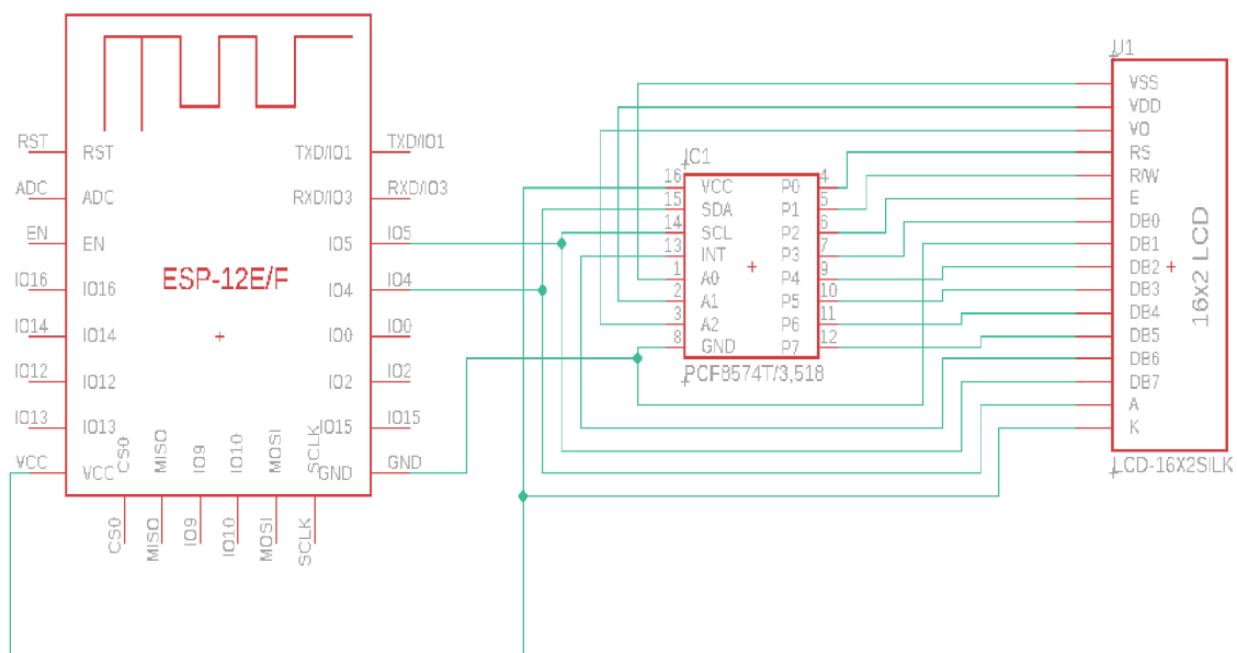
Obr. 5.3: zapojení displeje
