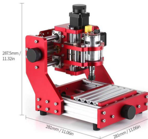
Obr. 2) Mini cnc 1310 [7]
