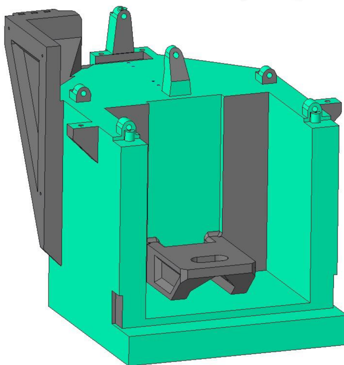
Obr. 16) Rám CNC frézky
