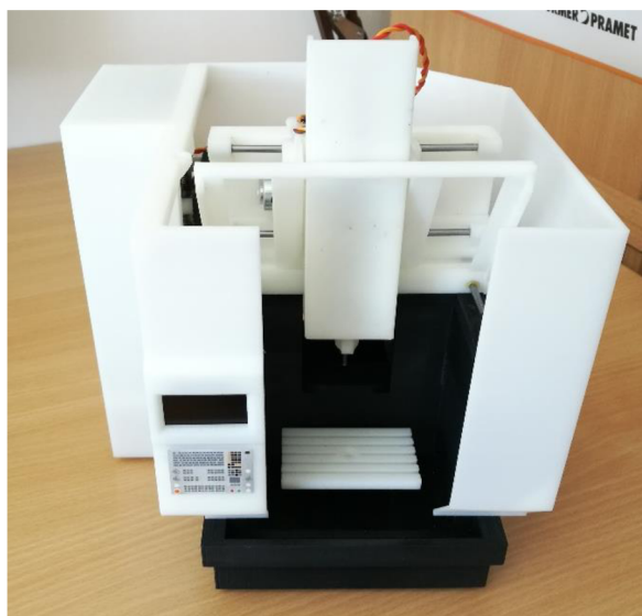
Obr. 37) Sestavený stroj
