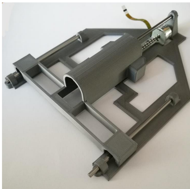
Obr. 28) První prototyp
