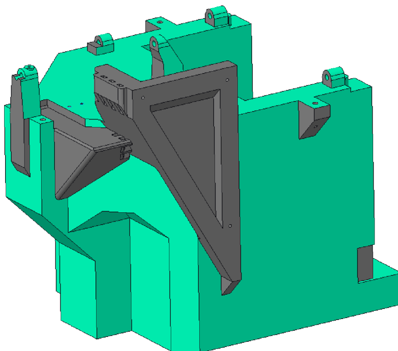
Obr. 18) rám s detailem na uchycení Arduina a kabeláže
