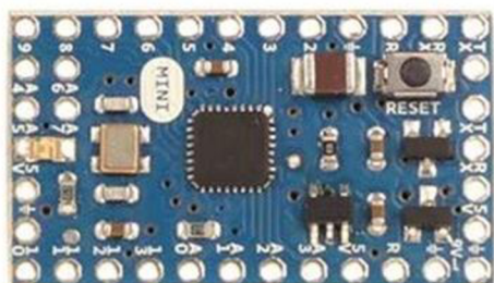
Obr. 7) Arduino Mini [13]
