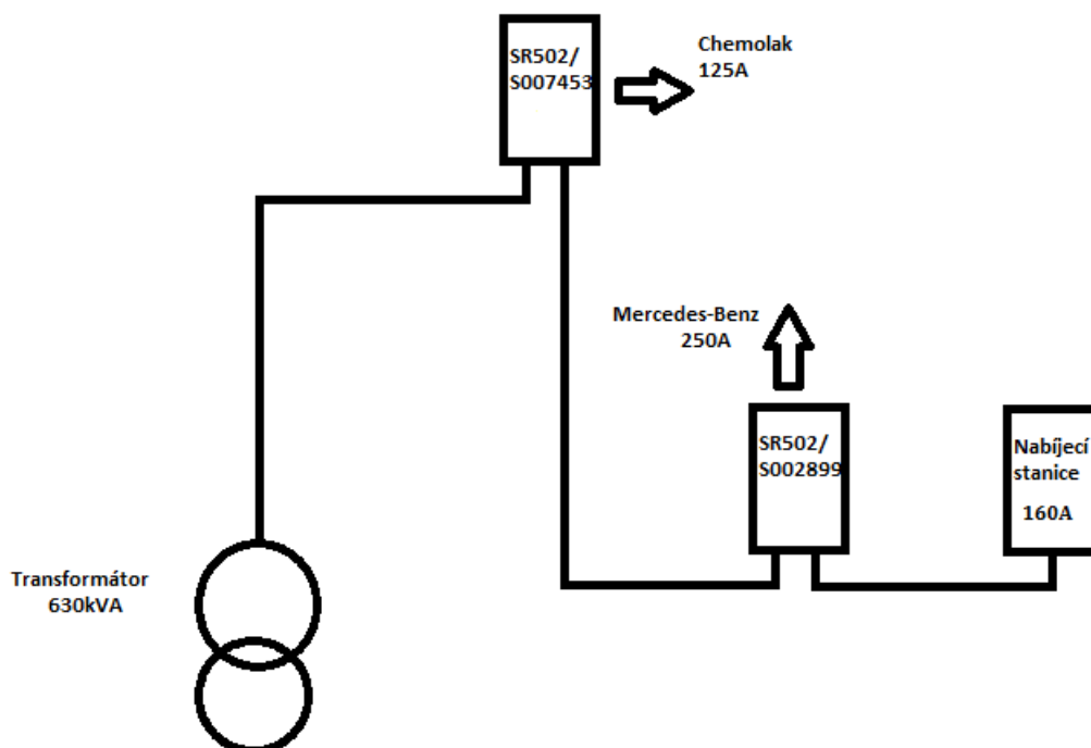
Obrázek 6-3 Schéma zapojení na již existující přívod
