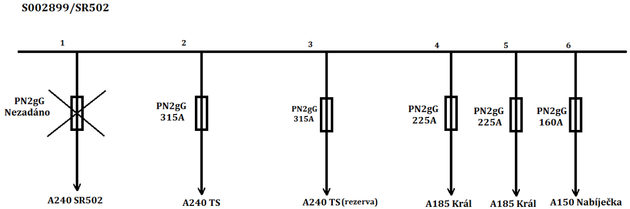
Obrázek 6-7 Detail skříně SR 502/S002899 pro případ 6.1.2
