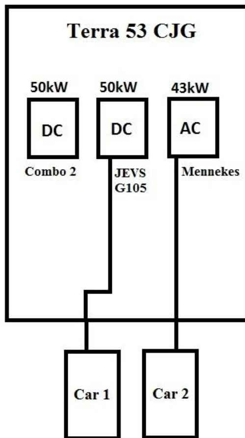
Obrázek 5-1 Schéma nabíjecí stanice
