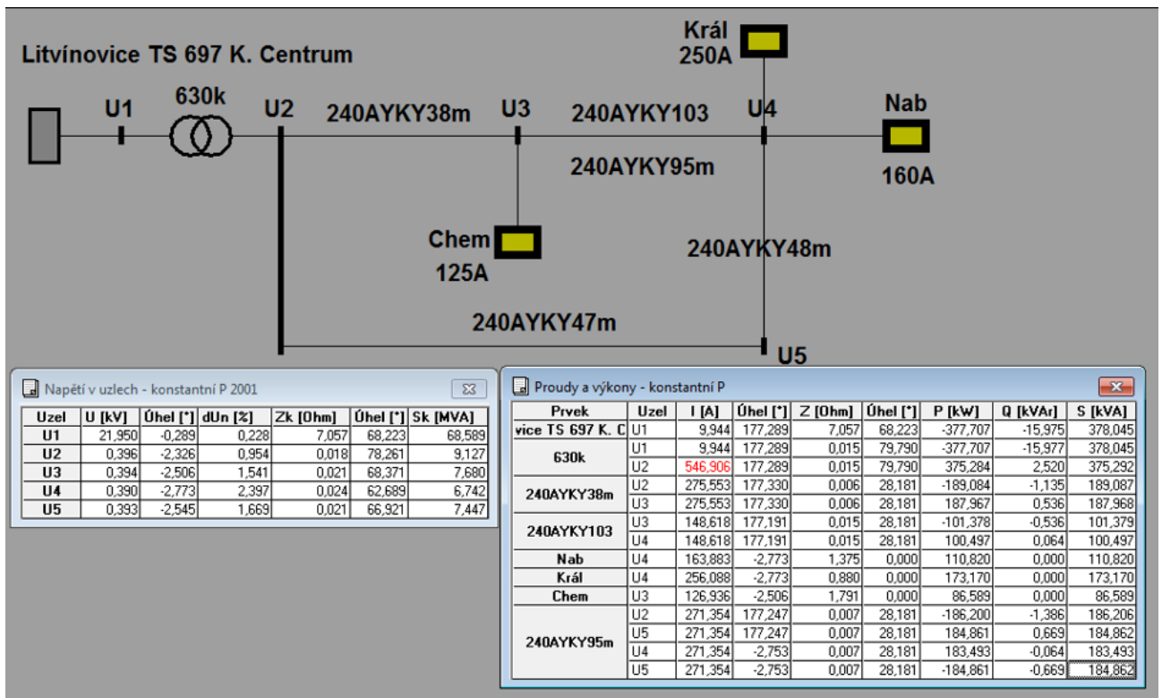
Obrázek 6-8 Simulace pro případ 6.1.2
