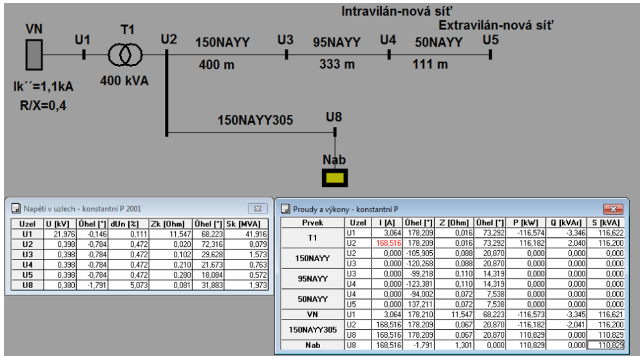
Obrázek 6-10 Simulace pro případ 6.3
