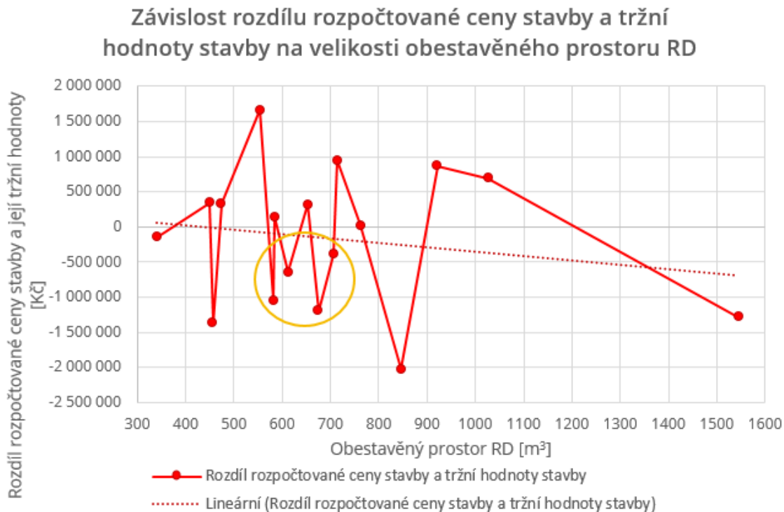
Obrázek č. 18 – Graf závislosti rozdílu rozpočtované ceny stavby a tržní hodnoty stavby na velikosti obestavěného prostoru RD s vyznačením ekonomicky nejméně efektivní oblasti
