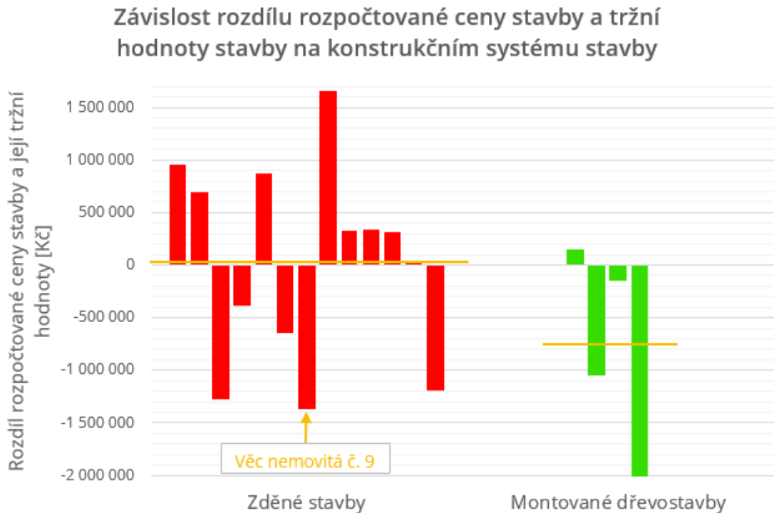
Obrázek č. 25 – Graf závislosti rozdílu rozpočtované ceny stavby a tržní hodnoty stavby na konstrukčním systému stavby s vyznačením VN č. 9
