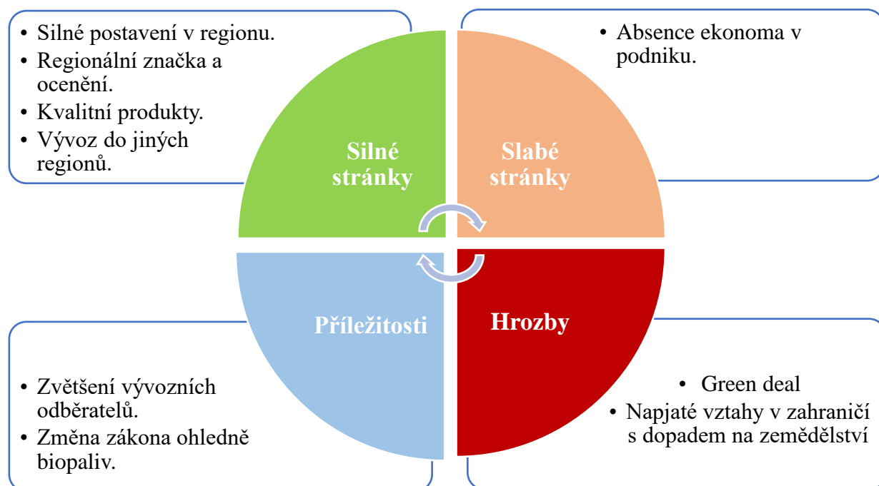
Obrázek 10: SWOT analýza
