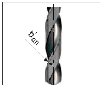
Obr. 2.7 Šířka fazetky
