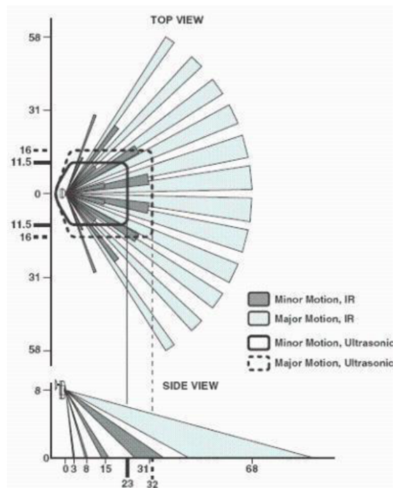
Obrázek 1: PIR detektor [3]
