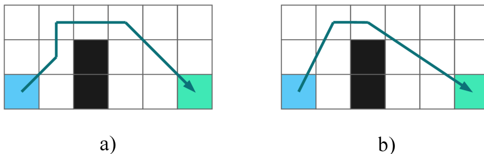
Obr. 25: (a) Cesta v mřížce (b) Any-angle cesta
