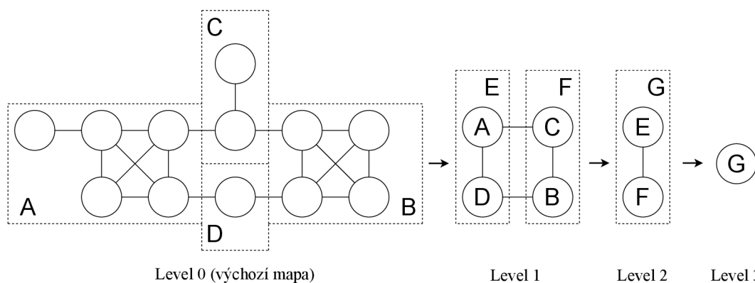
Obr. 16: Abstrakce prostřednictvím metody založené na klikách (podle [36, 38])
