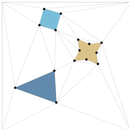
Obr. 8: Navigační síť
