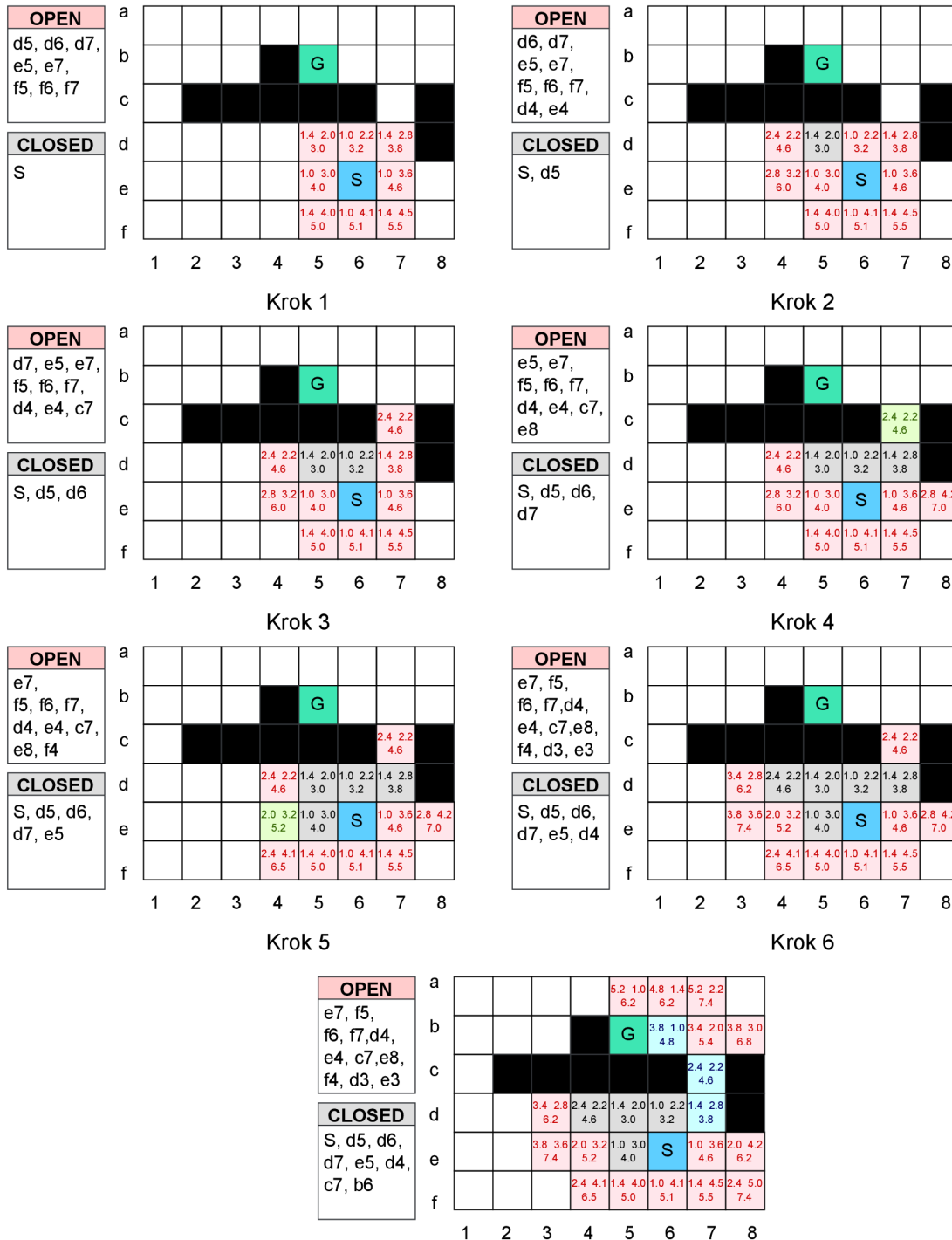
Obr. 14: Algoritmus A*
