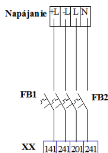
Obr. 2-3 Napájanie panelov
