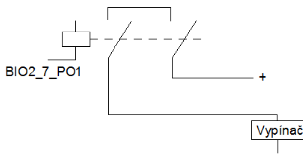
Obr. 3-4 Príklad zapojenia výkonového výstupu
