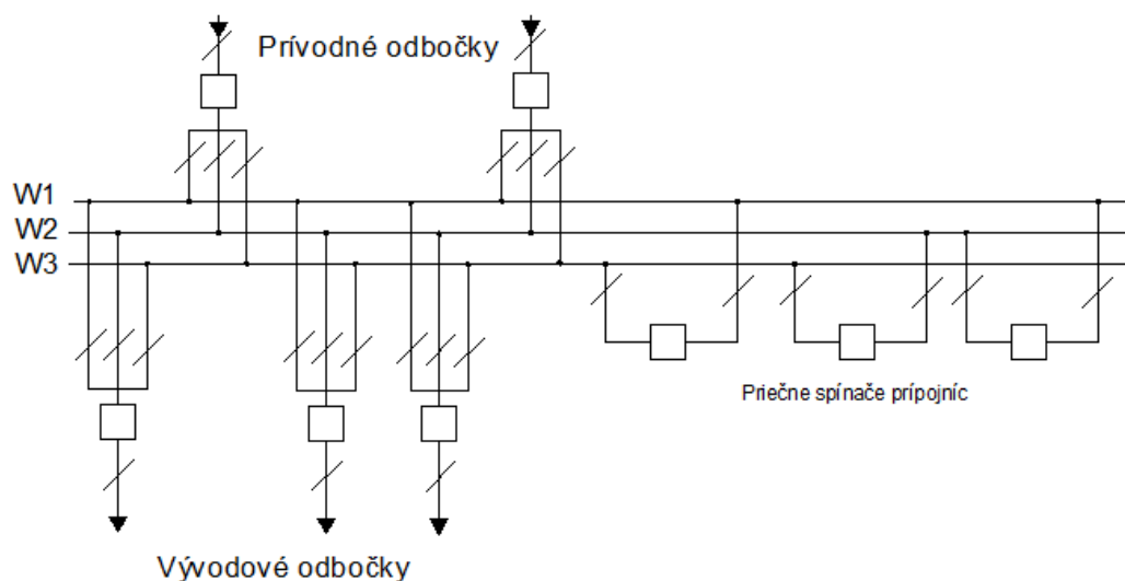
Obr. 4-3 Trojitý systém prípojnic
