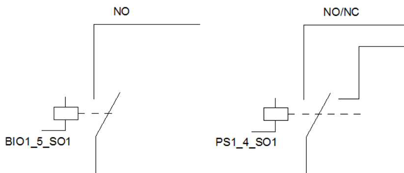
Obr. 3-5 Príklad zapojenia signalizačného výstupu
