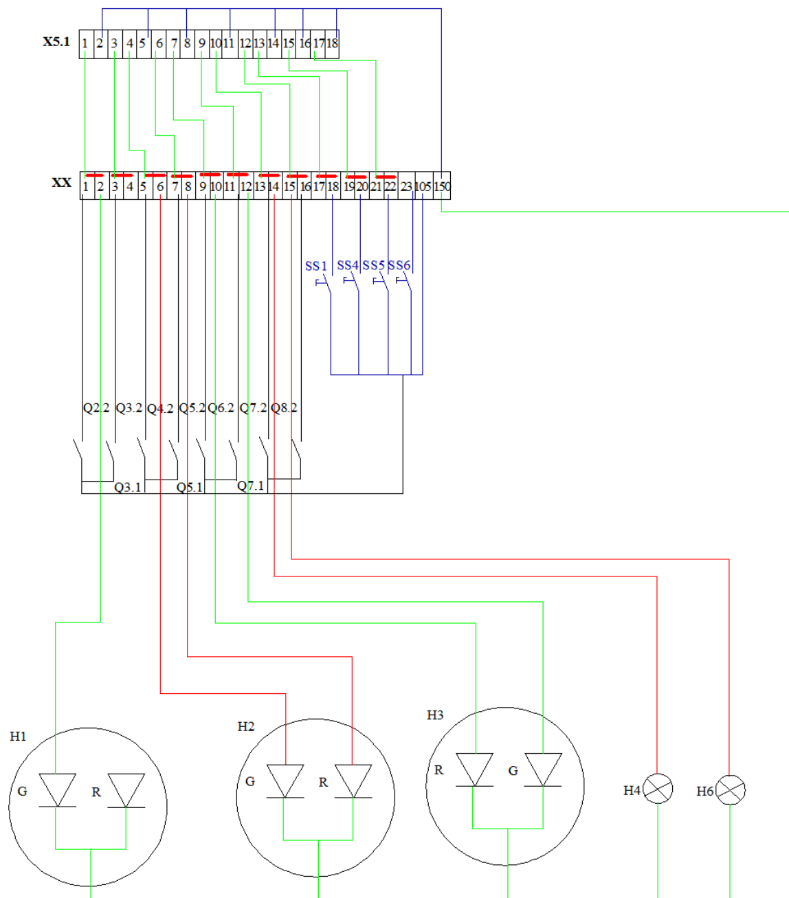
Obr.2-4 Vnútročné zapojenie skúšobných panelov (časť prvá)
