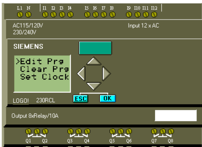
Obr. 2-6 Logický modul LOGO! 230RCL – prevzaté z [9]
