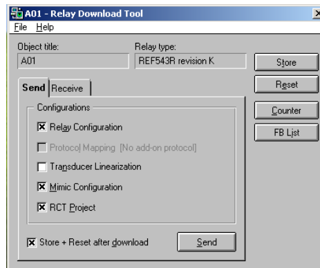
Obr. 5-9 Nahratie konfigurácie do ochranného terminálu
