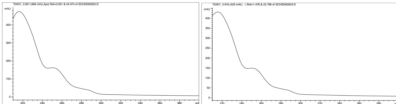
Obrázek 31: Absorpční UV spektrum vzorku CH 2 (vlevo) a CH 3 (vpravo).
