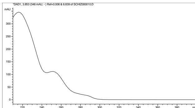
Obrázek 30: Absorpční UV spektrum vzorku CZ 3 (vlevo) a CH 1 (vpravo).
