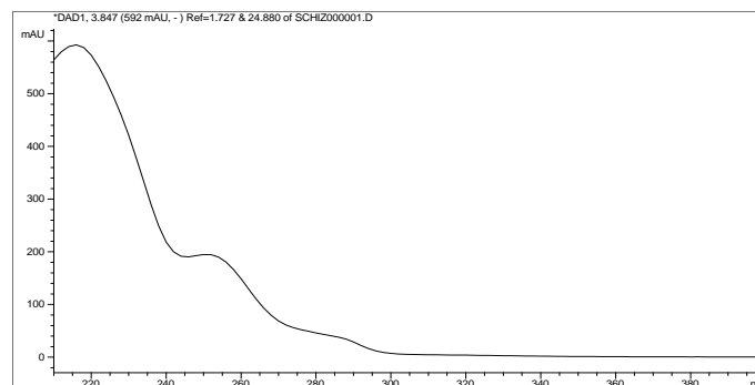
Obrázek 30: Absorpční UV spektrum vzorku CZ 3 (vlevo) a CH 1 (vpravo).
