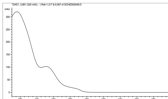
Obrázek 29: Absorpční UV spektrum vzorku CZ 1 (vlevo) a CZ 2 (vpravo).
