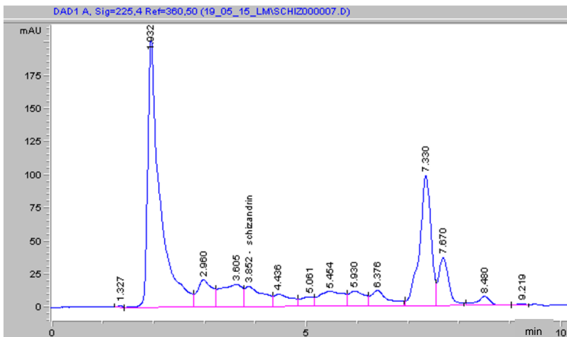
Obrázek 14: Chromatogram vzorku 1 - Sox CH řaděné
