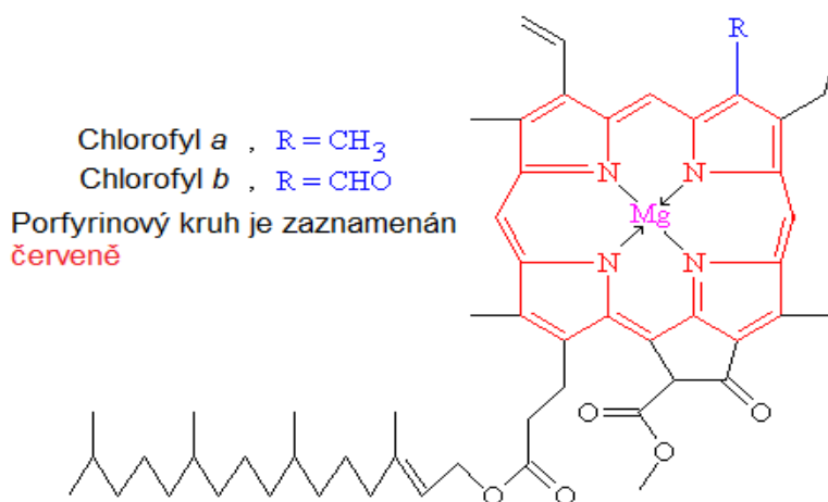
Obrázek 8: Struktura chlorofylu a a chlorofylu b
