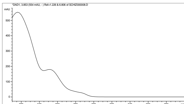
Obrázek 29: Absorpční UV spektrum vzorku CZ 1 (vlevo) a CZ 2 (vpravo).
