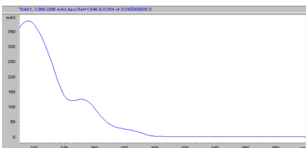
Obrázek 27: Absorpční UV spektrum standardu schizandrinu A (vlevo) a Sox CH neřaděného (vpravo).
