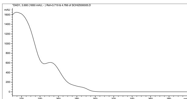
Obrázek 27: Absorpční UV spektrum standardu schizandrinu A (vlevo) a Sox CH neřaděného (vpravo).
