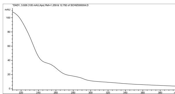
Obrázek 27: Absorpční UV spektrum standardu schizandrinu A (vlevo) a Sox CH neřaděného (vpravo).
