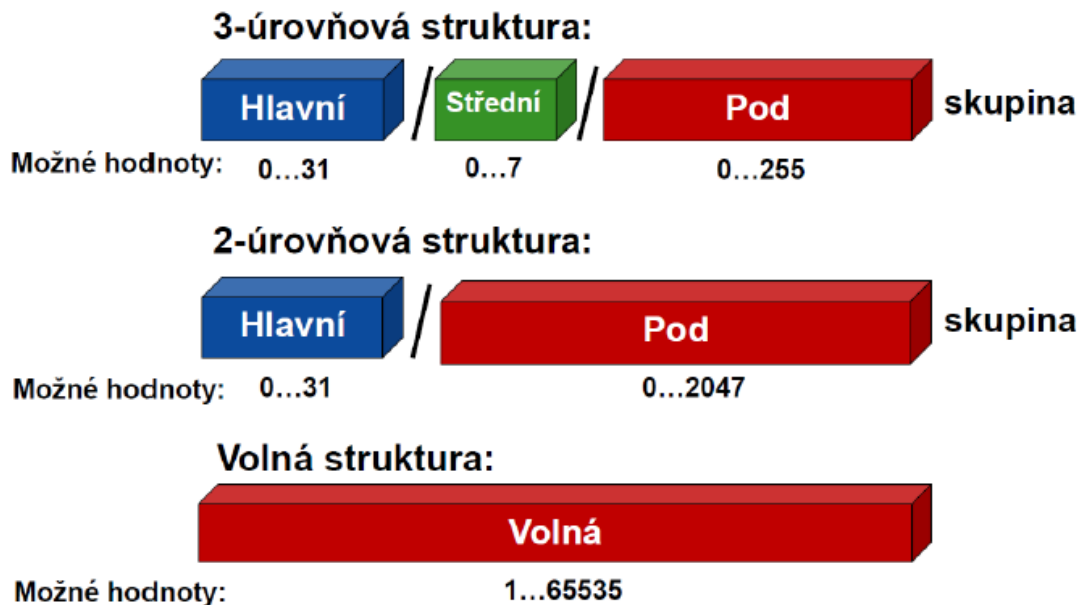
Obrázek 2 – Možné struktury skupinových adres [3]
