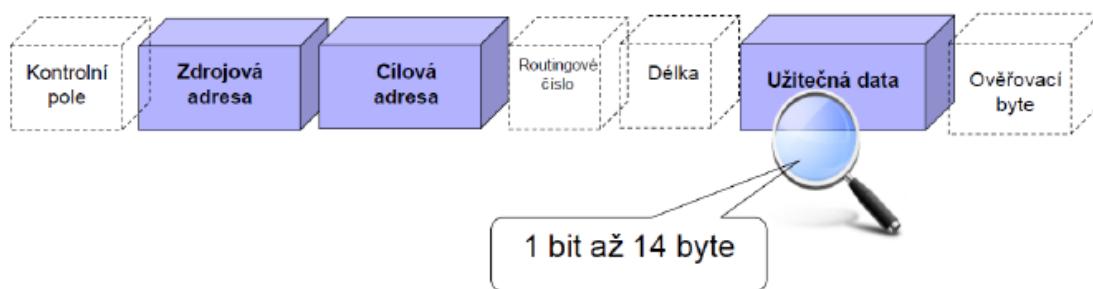
Obrázek 3 – Telegram na sběrnici [3]
