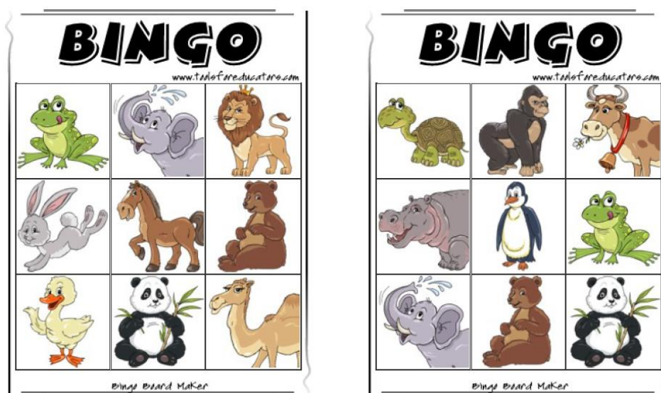
Obrázek 8 – Bingo cards 7
