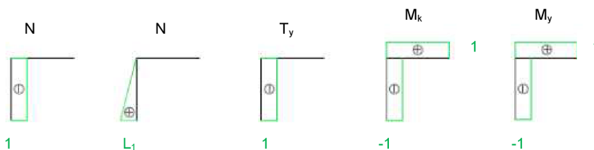
Obr. 27 Zaťaženia ložísk virtuálnymi silami + VVÚ od nich spôsobené
