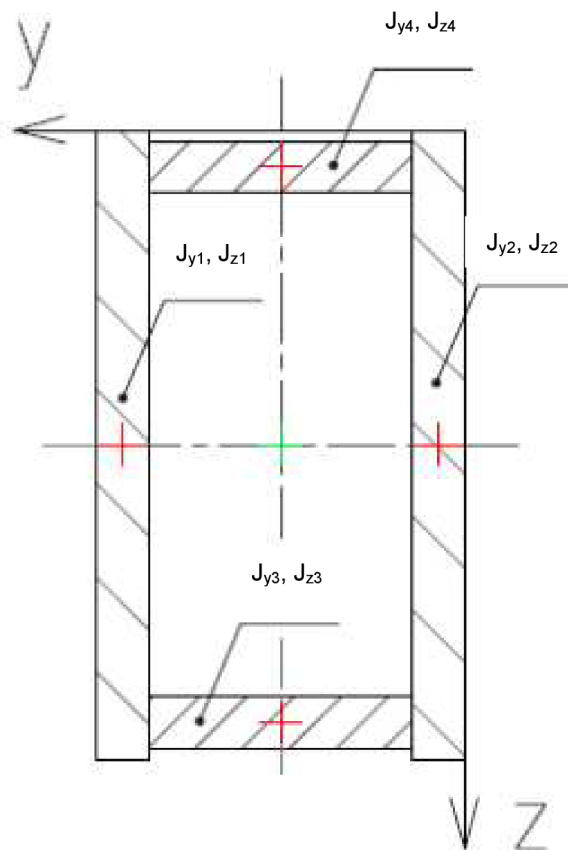
Obr. 21 Osovú kvadratické momenty priečného prierezu rámu
