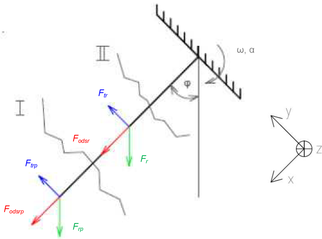
Obr. 5 VVÚ a súradnicový systém pre ľavicové rameno pohybujúce sa maximálnym uhlovým zrýchlením
