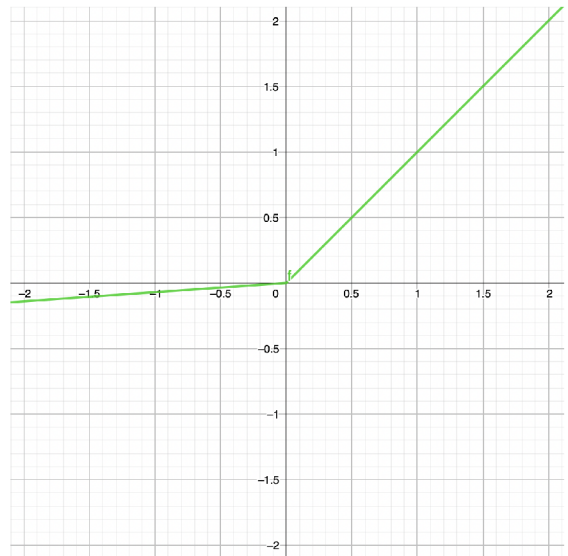
Obr. 1.6: Průběh aktivační funkce LReLU
