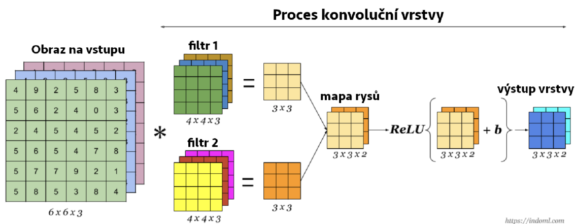
Obr. 1.9: Architektura a proces konvoluční vrstvy, převzato z [7]
