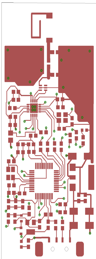
Obrázek 4.16: DPS - vrchní strana
