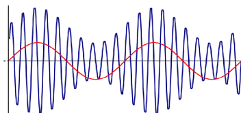
Obrázek 6.3: Amplitudová modulace harmonického signálu
