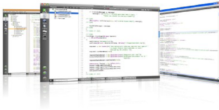
Obrázek 5.3: Qt Creator
