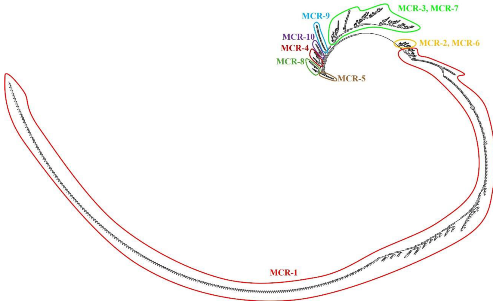
Obrázek 7: Fylogenetický strom získaný porovnáním 800 enzymů MCR pomocí Geneious PhyML. Jednotliví zástupci rodin MCR jsou zvýrazněni barevnými čarami.
