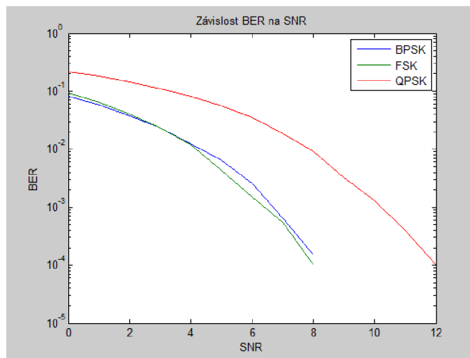
Obr. 4.11: graf závislosti modulací BPSK, FSK a QPSK na chybovosti BER
