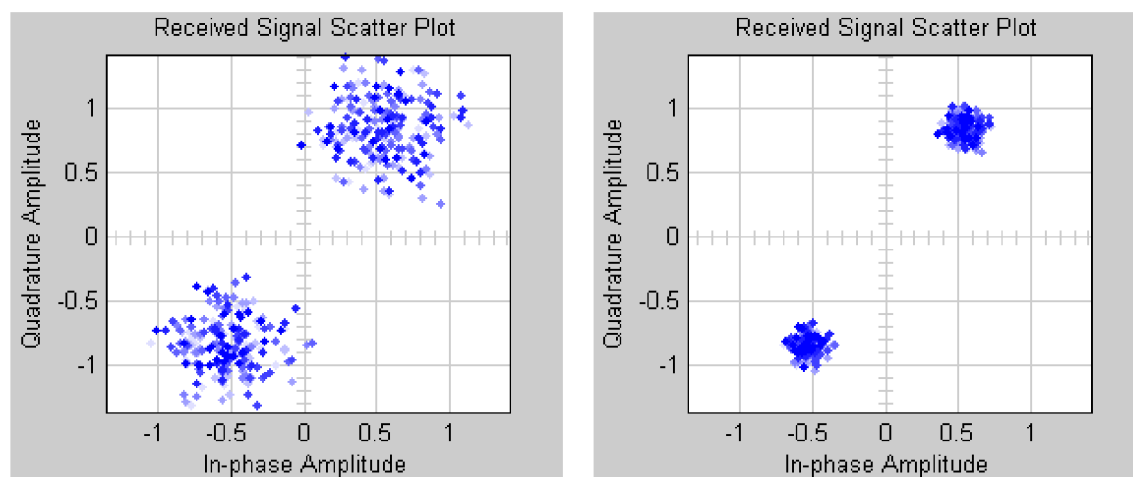
Obr. 4.4: konstelační diagram modulace BPSK při SNR a) 10 dB b) 20 dB
