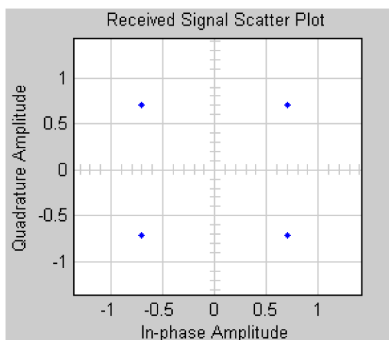
Obr. 4.7: konstelační diagram modulace QPSK před kanálem
