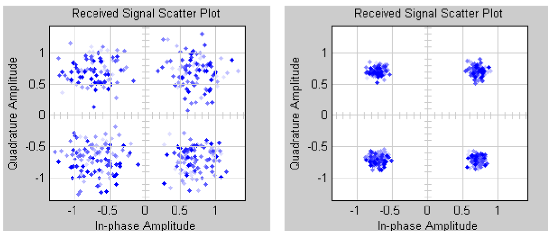
Obr. 4.8: konstelační diagram modulace QPSK při SNR a) 10 dB b) 20 dB
