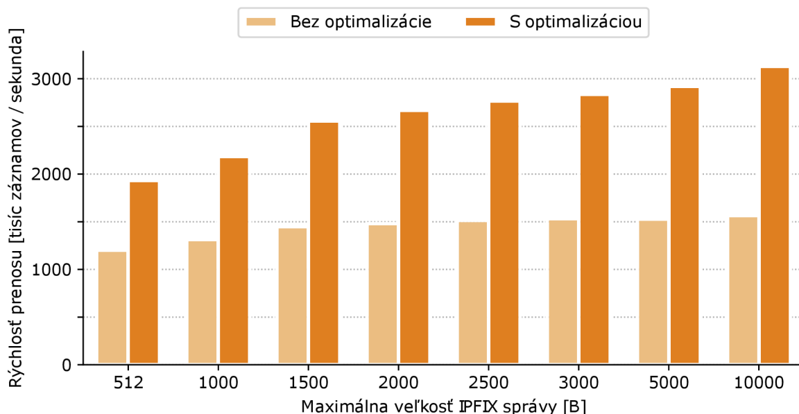
Obr. 5.6: Porovnanie výkonnosti kolektoru s ukázkovým modulom pri použití optimalizácie
