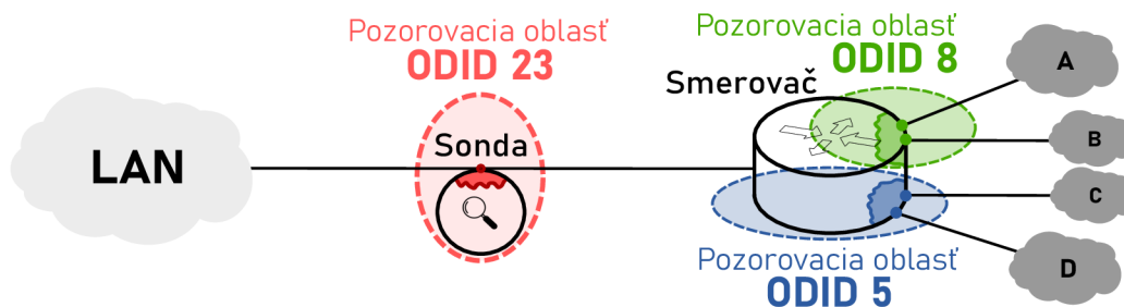
Obr. 2.3: Príklady pozorovacích oblastí architektúry NetFlow/IPFIX
